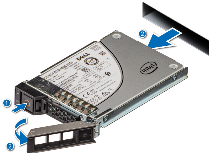
Ilustración 35. Extracción de un portaunidades
