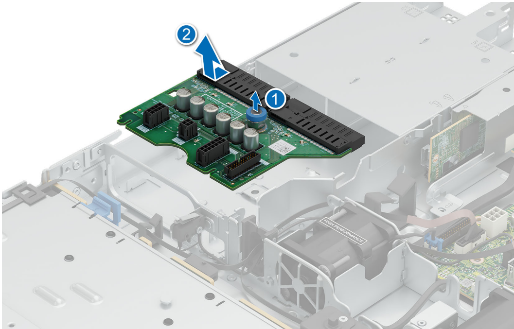
Ilustración 75. Extracción de la PIB
