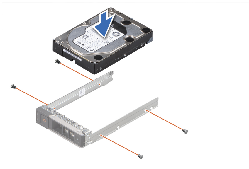
Ilustración 37. Instalación de una unidad en el portaunidades
