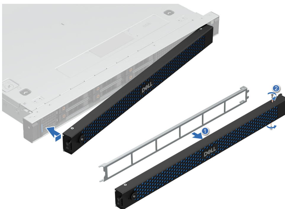
Ilustración 87. Instalación del bisel del filtro
