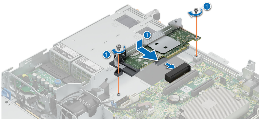
Ilustración 66. Instalación de la tarjeta PERC interna
