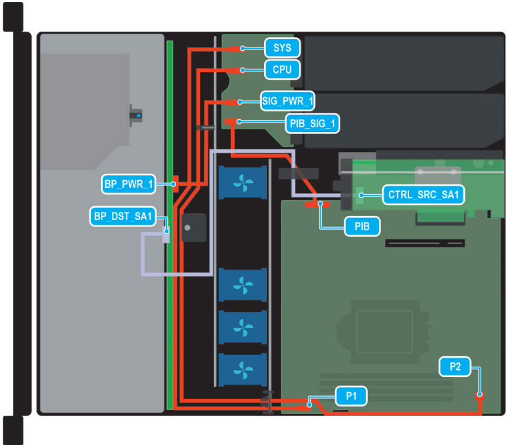
Ilustración 30. Configuración 2: 4 de SAS/SATA de 3,5 pulgadas y tarjeta PERC interna
