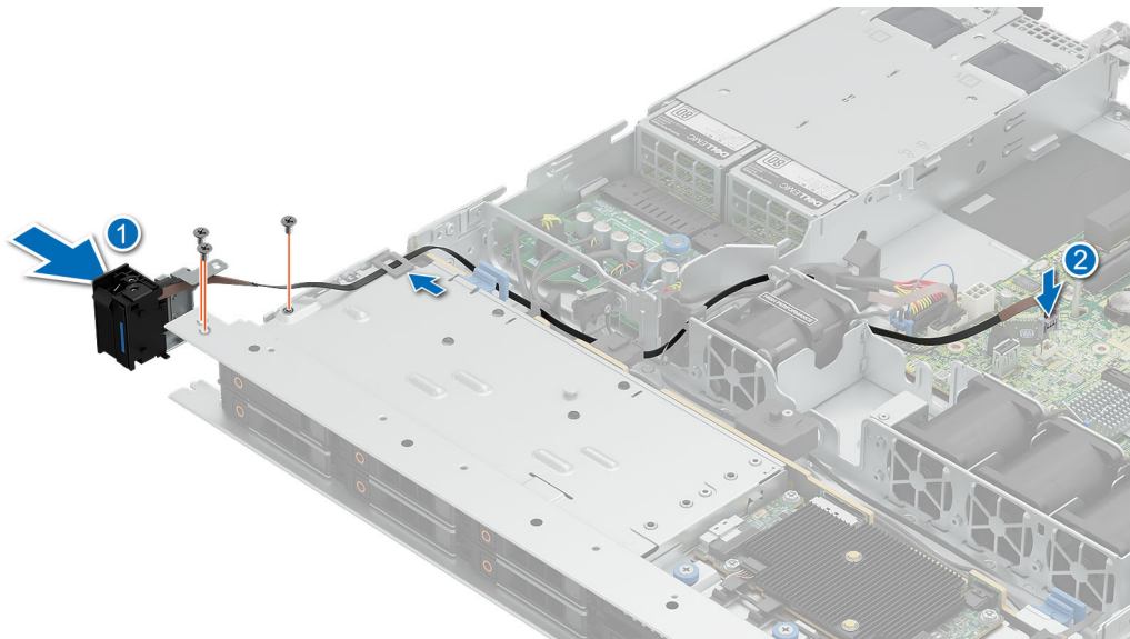
Ilustración 82. Extracción del panel de control izquierdo
