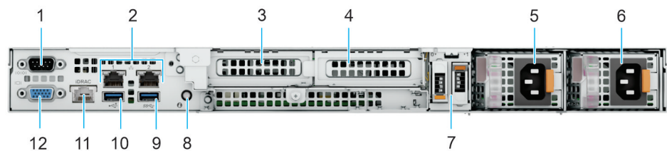
Ilustración 3. Vista posterior del sistema
