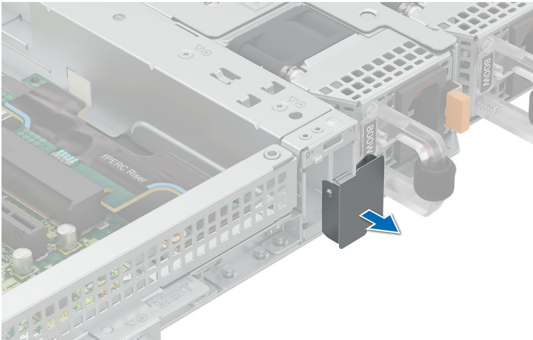
Ilustración 84. Extracción del módulo de BOSS-N1 de relleno
