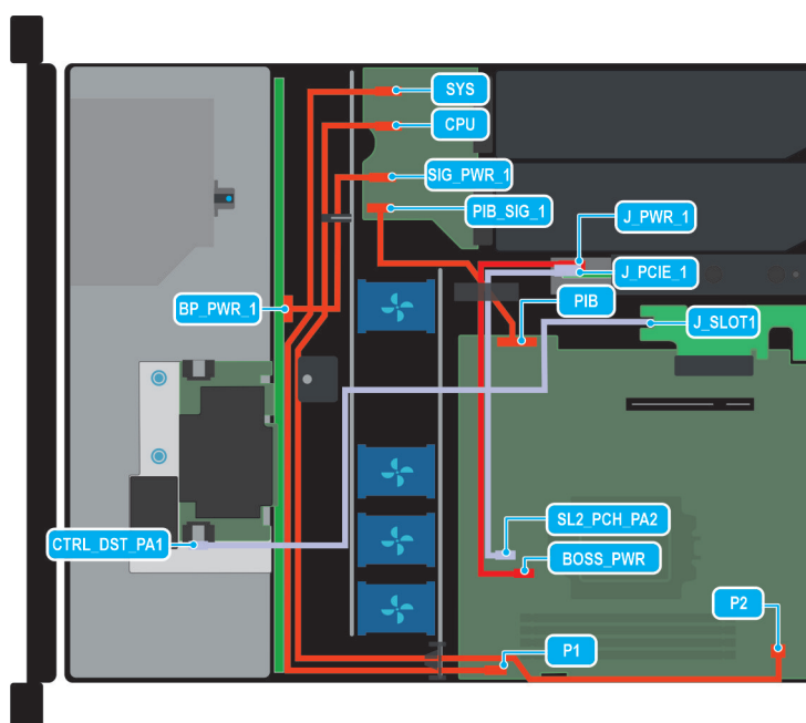
Ilustración 29. Configuración 1: SAS/SATA de 4 x 3,5 pulgadas y fPERC con BOSS N1 (opcional)
