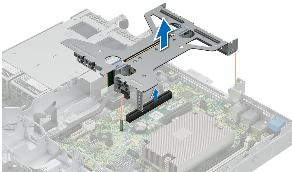
Ilustración 53. Extracción de la tarjeta elevadora
