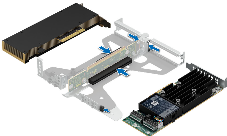
Ilustración 52. Instalación de una tarjeta de expansión en la tarjeta elevadora
