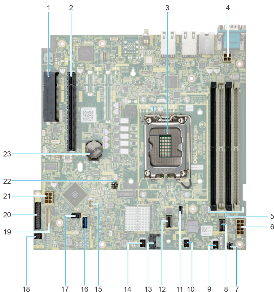
Ilustración 88. Puentes y conectores de la tarjeta madre del sistema
