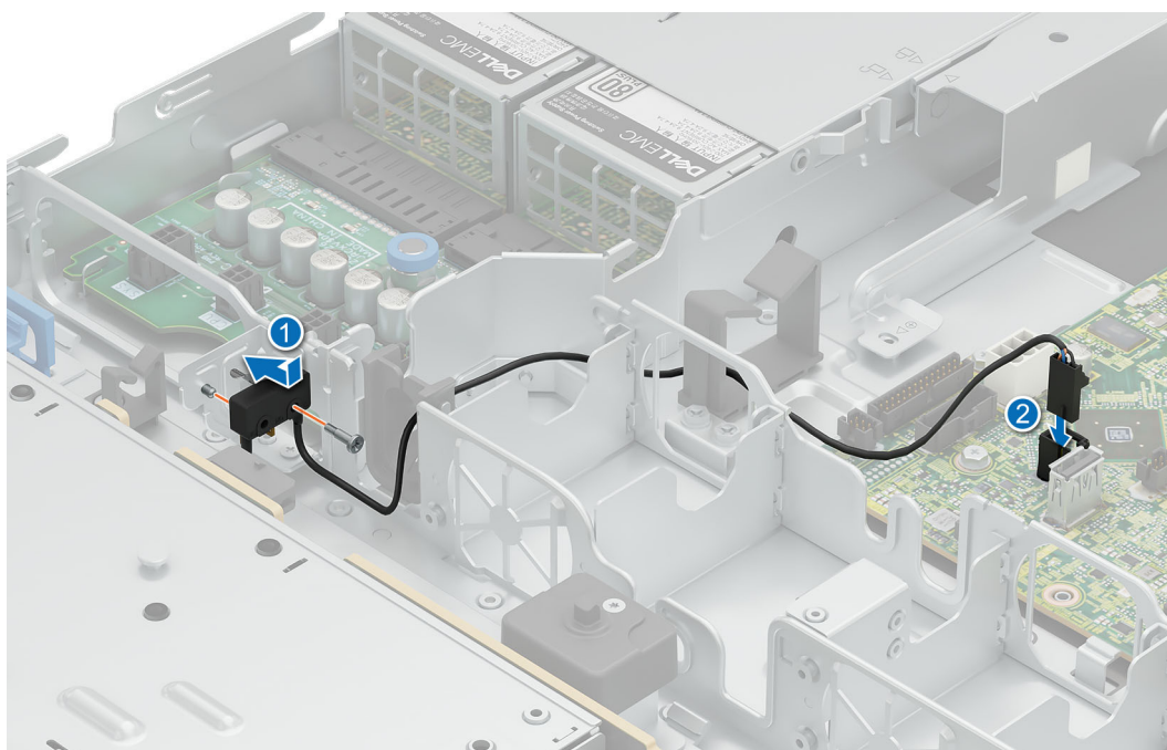
Ilustración 23. Instalación del interruptor de intrusiones
