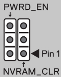
Ilustración 8. Configuración de los puentes
