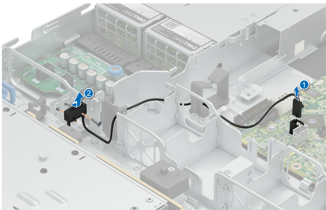
Ilustración 22. Extracción del interruptor de intrusiones
