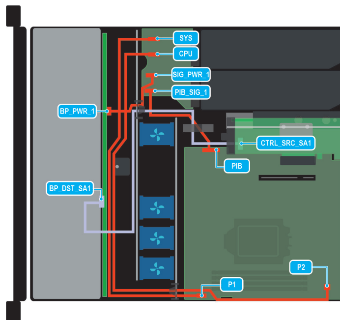
Ilustración 32. Configuración 4: 8 SAS/SATA de 2,5 pulgadas y tarjeta PERC interna
