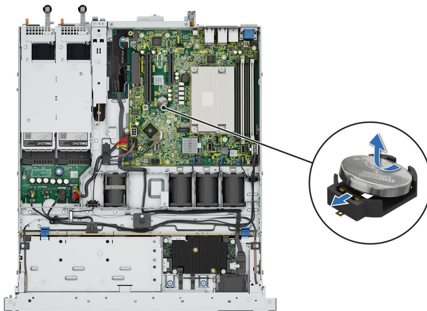
Ilustración 63. Extracción de la batería del sistema
