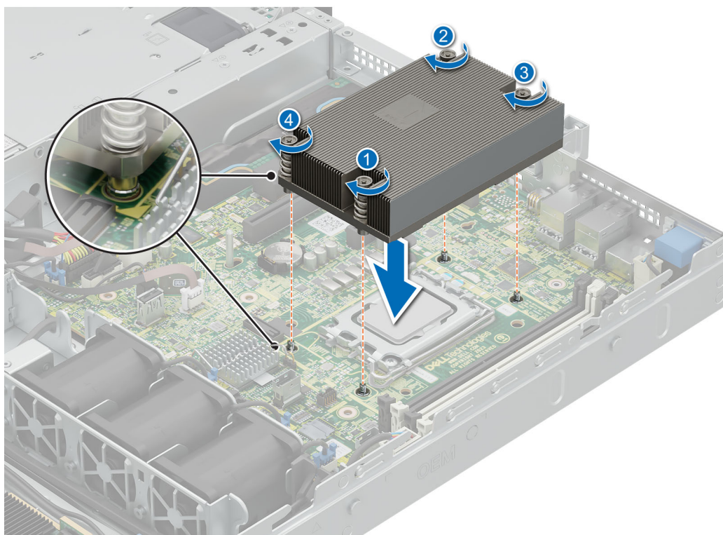
Ilustración 49. Instalación del disipador de calor
