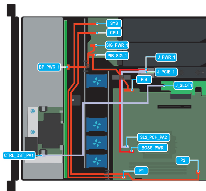
Ilustración 31. Configuración 3: tarjeta fPERC y SAS/SATA de 8 x 2,5 pulgadas con BOSS N1 opcional
