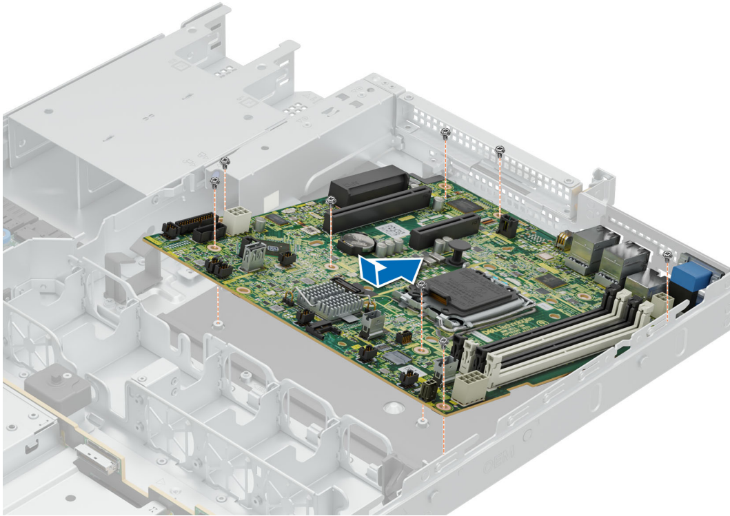
Ilustración 78. Instalación de la tarjeta madre
