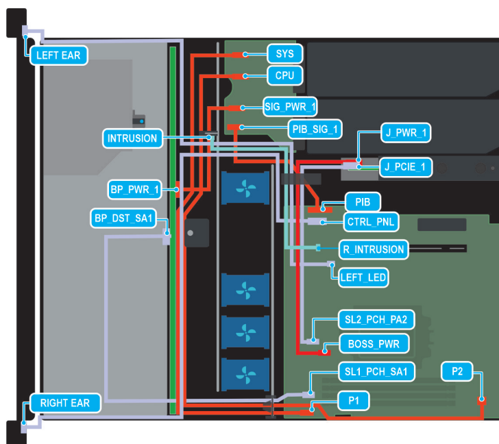
Ilustración 28. Configuración 0: SATA de 4 x 3,5 pulgadas con BOSS N1 (opcional)
