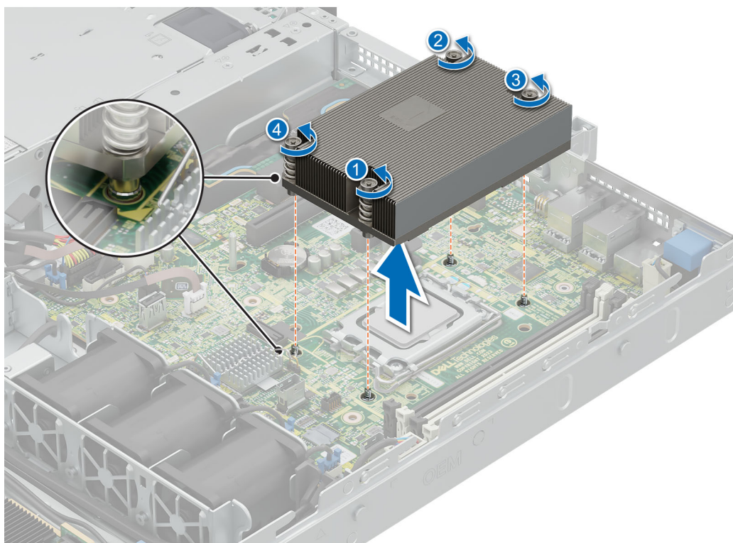
Ilustración 44. Extracción del módulo del disipador de calor
