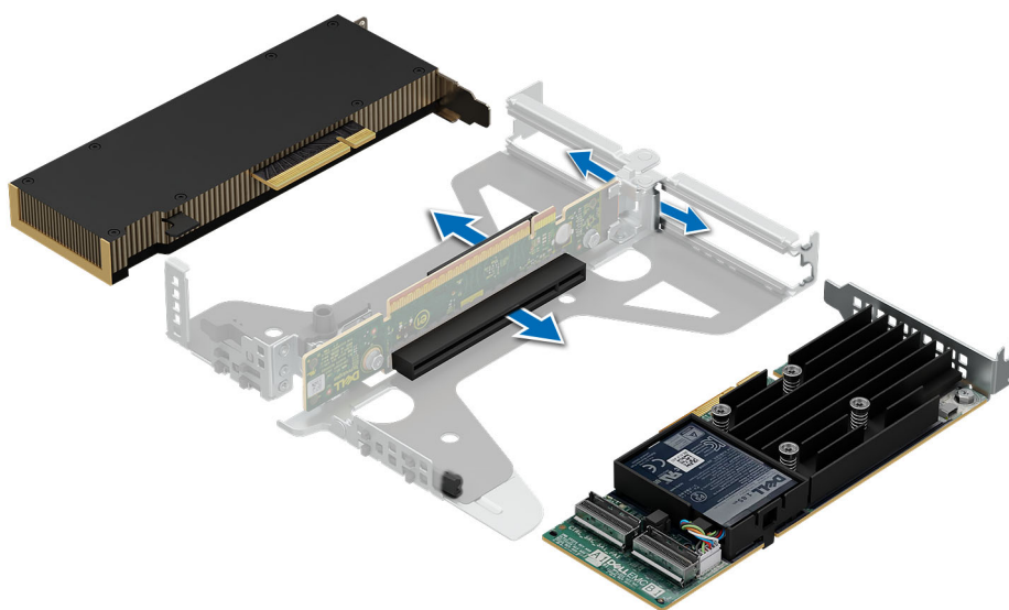
Ilustración 50. Extracción de una tarjeta de expansión de la tarjeta elevadora
