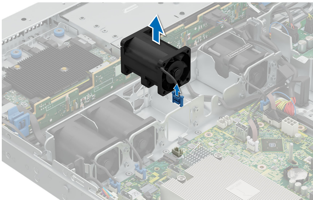
Ilustración 20. Extracción del ventilador de enfriamiento
