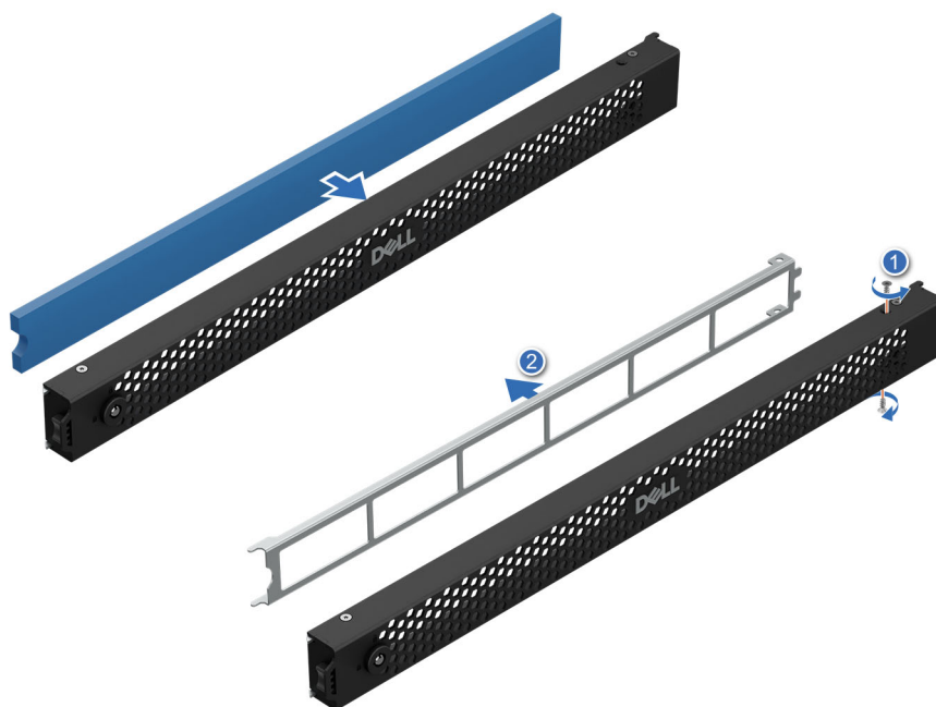
Ilustración 86. Instalación del filtro
