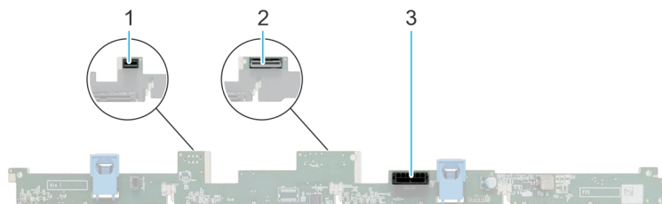
Ilustración 25. Backplane de 4 unidades SAS/SATA/SSD de 3,5 pulgadas
