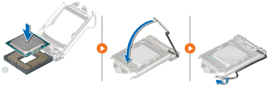
Ilustración 46. Instalación del gancho de retención
