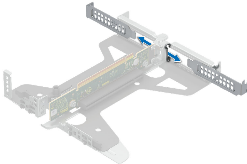
Ilustración 51. Extracción del soporte de relleno de la tarjeta elevadora
