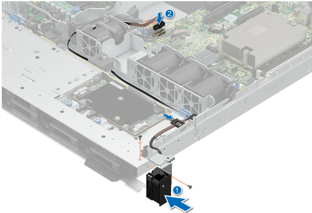
Ilustración 81. Instalación del panel de control derecho
