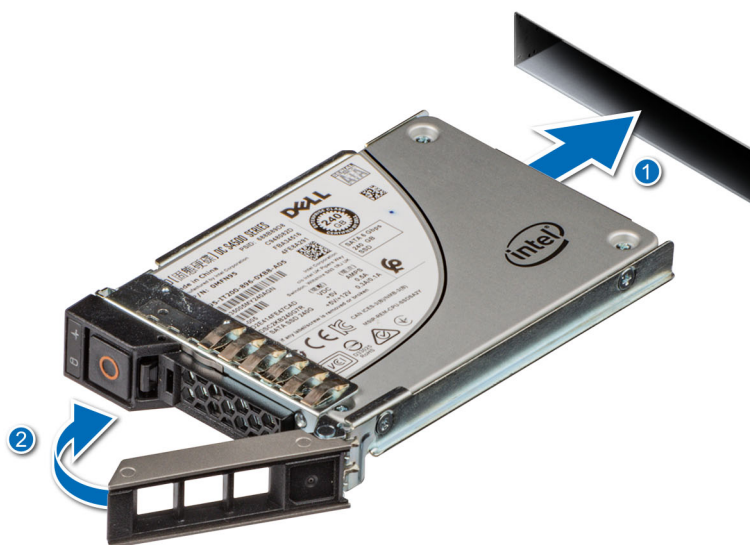
Ilustración 38. Instalación de un portaunidades
