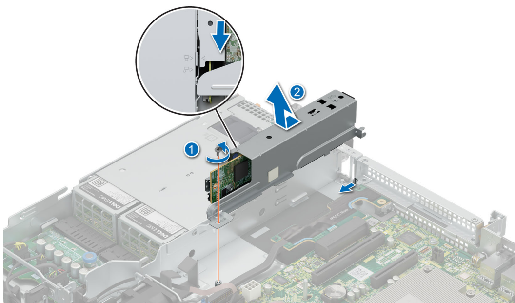
Ilustración 56. Extracción de la canastilla de BOSS N1
