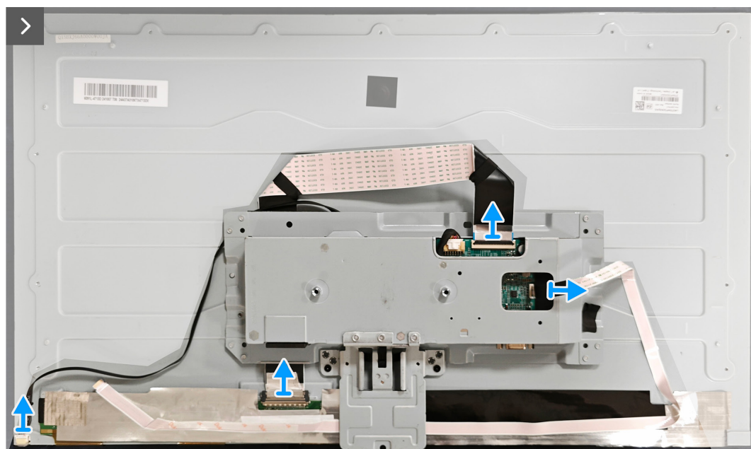
Figura 15. Retirar la protección metálica
