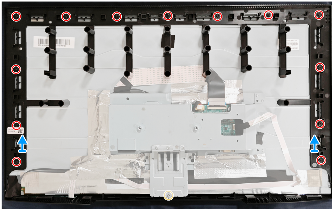
Figura 13. Retirar el marco central
