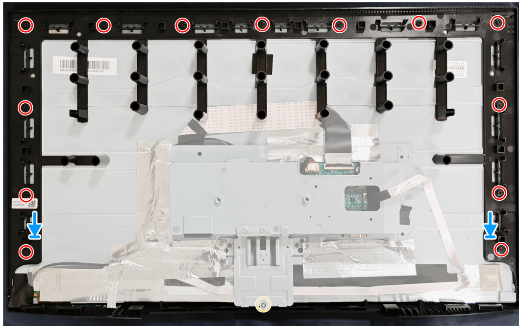
Figura 14. Instalar el marco central
