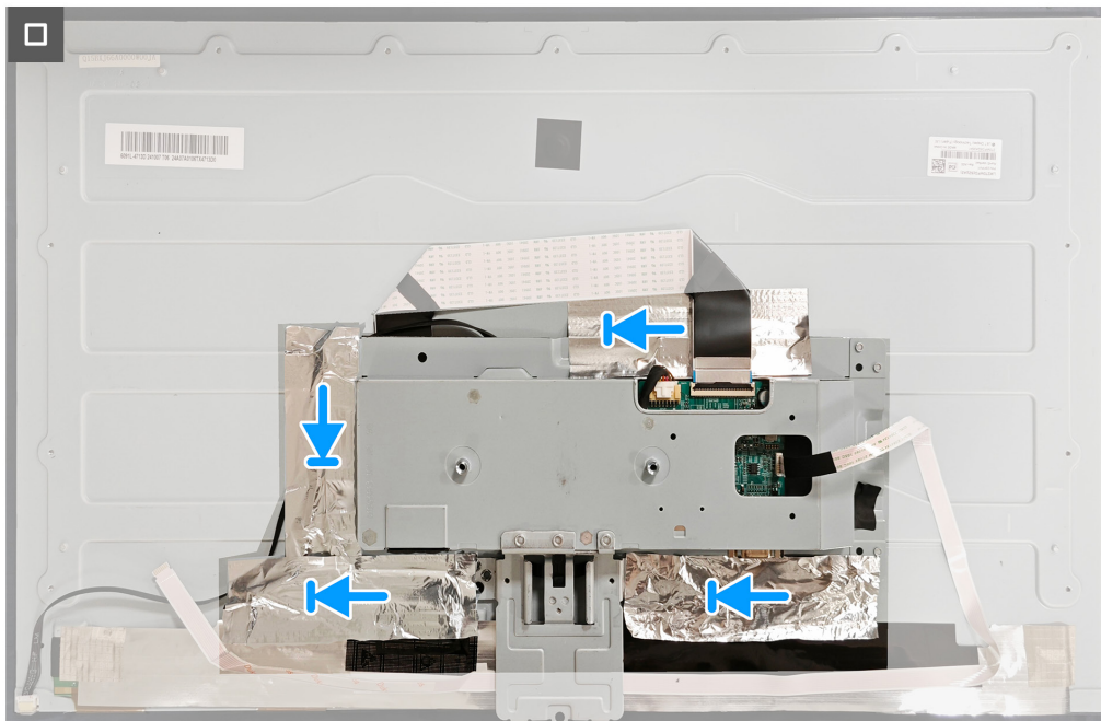
Figura 18. Instalar la protección metálica
