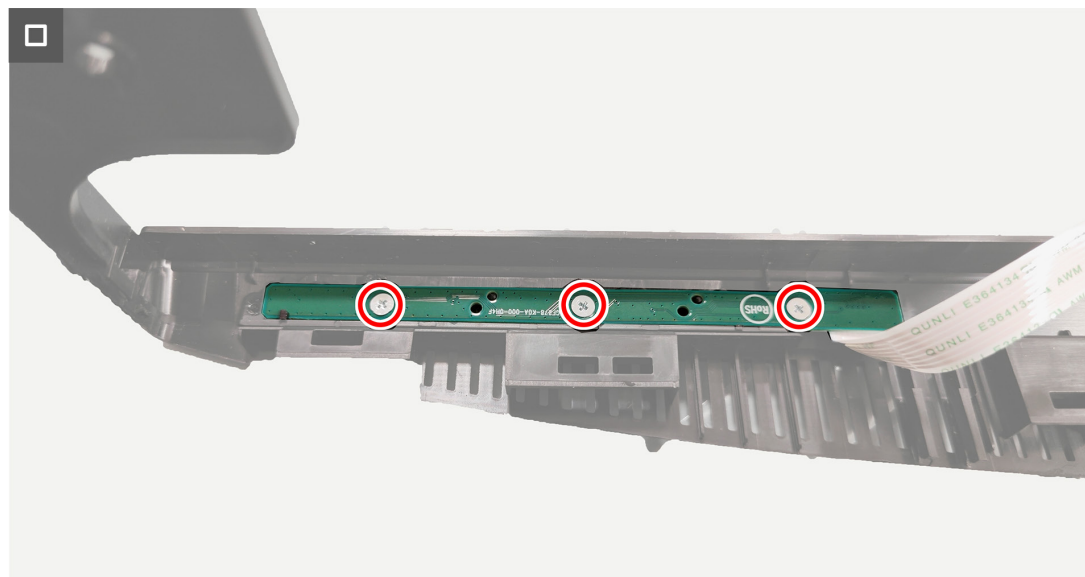
Figura 20. Instalar la placa del teclado
