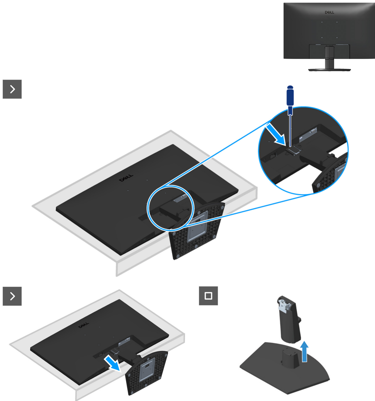
Figura 9. Retirar el pedestal
