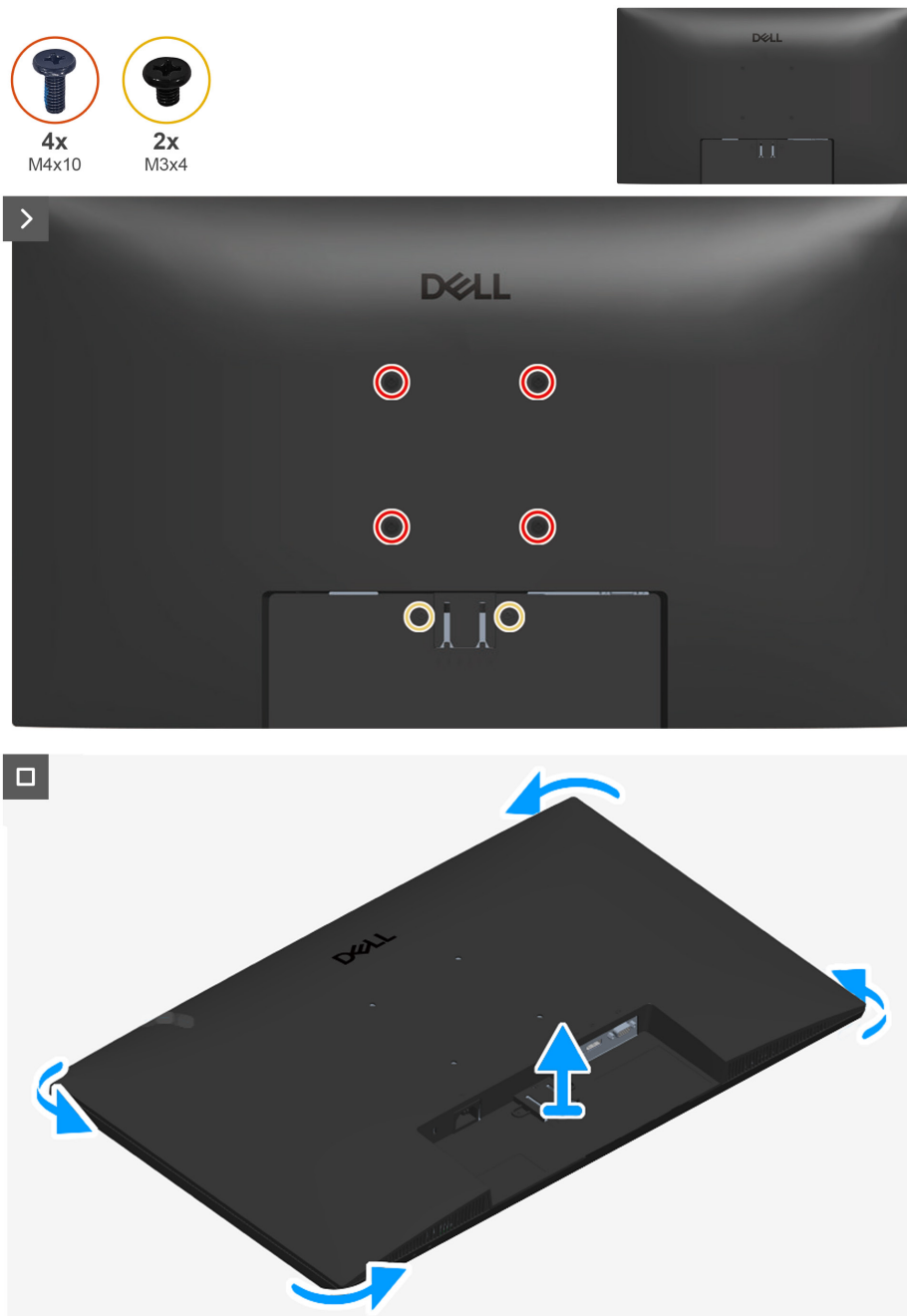
Figura 11. Retirar la cubierta posterior
