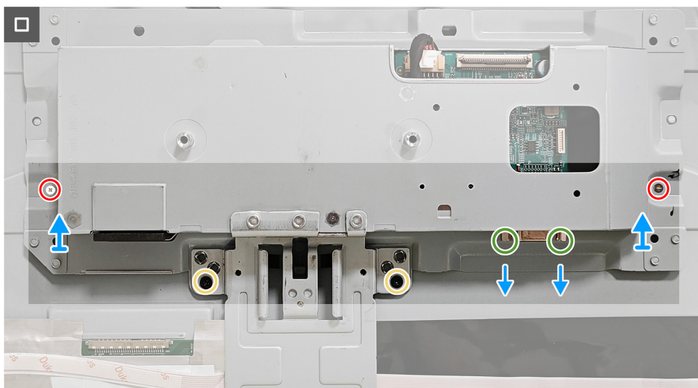
Figura 16. Retirar la protección metálica
