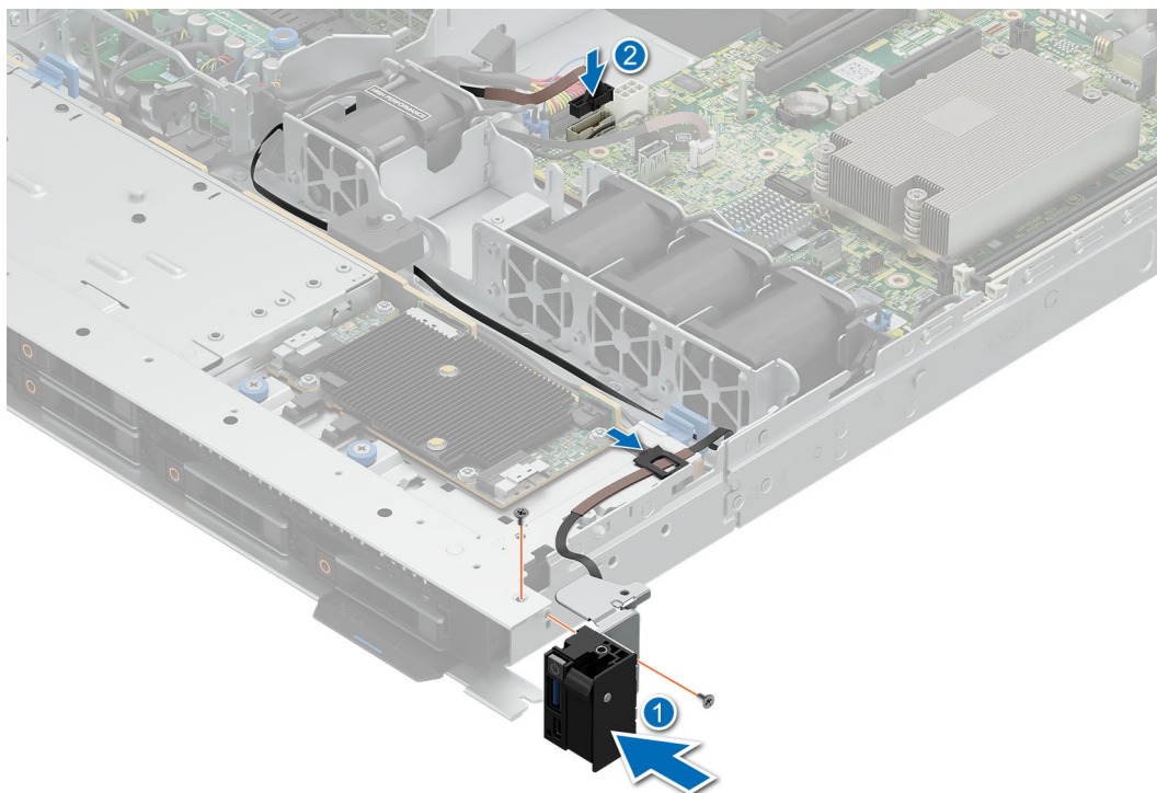
Ilustración 81. Instalación del panel de control derecho
