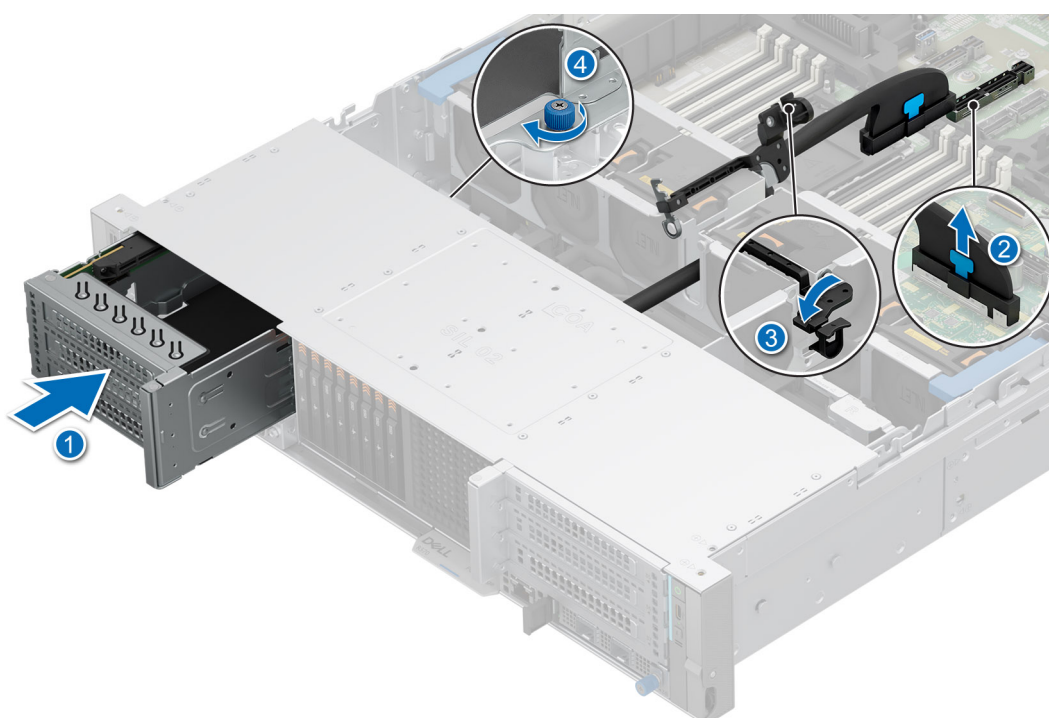
Ilustración 139. Instalación de la tarjeta elevadora para tarjetas de expansión frontal 1
