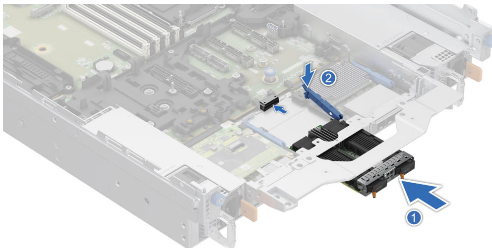
Ilustración 227. Instalación del módulo BOSS-N1 DC-MHS
