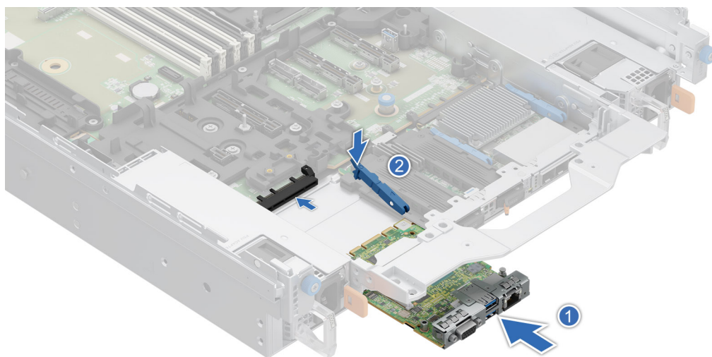
Ilustración 241. Instalación de la placa DC-SCM
