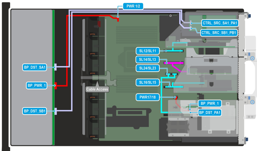
Ilustración 97. C04-02 Configuración de cable 20: 12 x 3,5 pulgadas (SAS/SATA)
