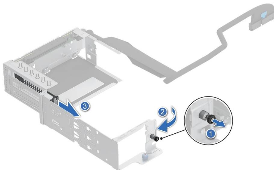
Ilustración 143. Extracción del soporte de relleno
