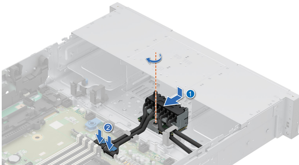
Ilustración 74. Instalación del módulo de backplane EDSFF E3.S
