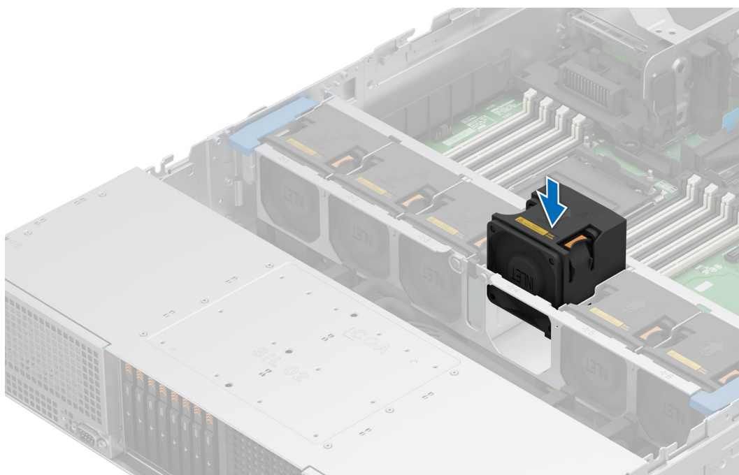
Ilustración 39. Instalación de un ventilador de enfriamiento
