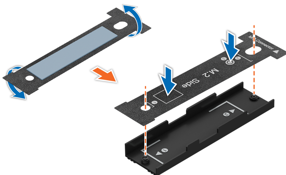
Ilustración 210. Instalación de la nueva almohadilla térmica dentro de la cubierta superior
