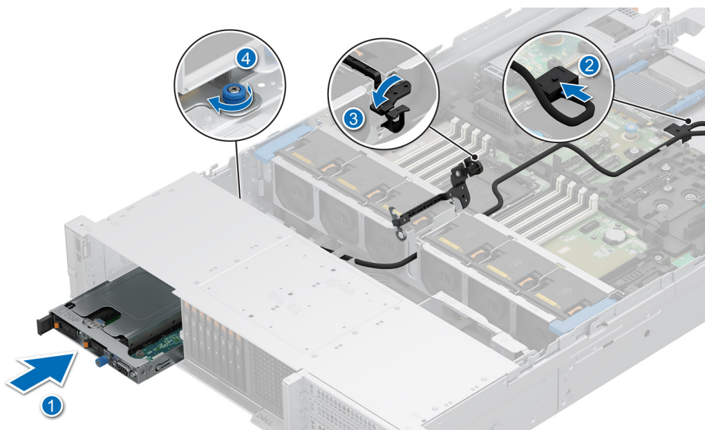
Ilustración 136. Instalación de la tarjeta elevadora para tarjetas de expansión frontal 2
