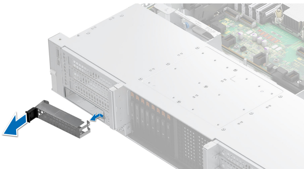
Ilustración 220. Extracción de un soporte de relleno para la controladora BOSS-N1 DC-MHS
