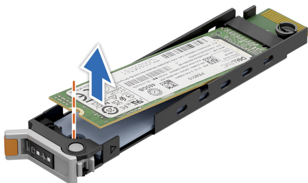
Ilustración 185. Extracción del módulo de SSD NVMe M.2
