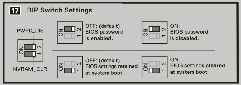
Ilustración 19. Configuración del switch de DIP
