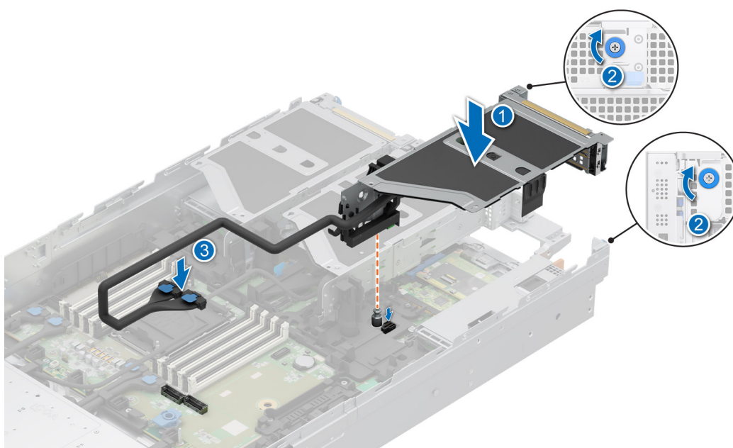
Ilustración 155. Instalación de la tarjeta elevadora para tarjetas de expansión 1
