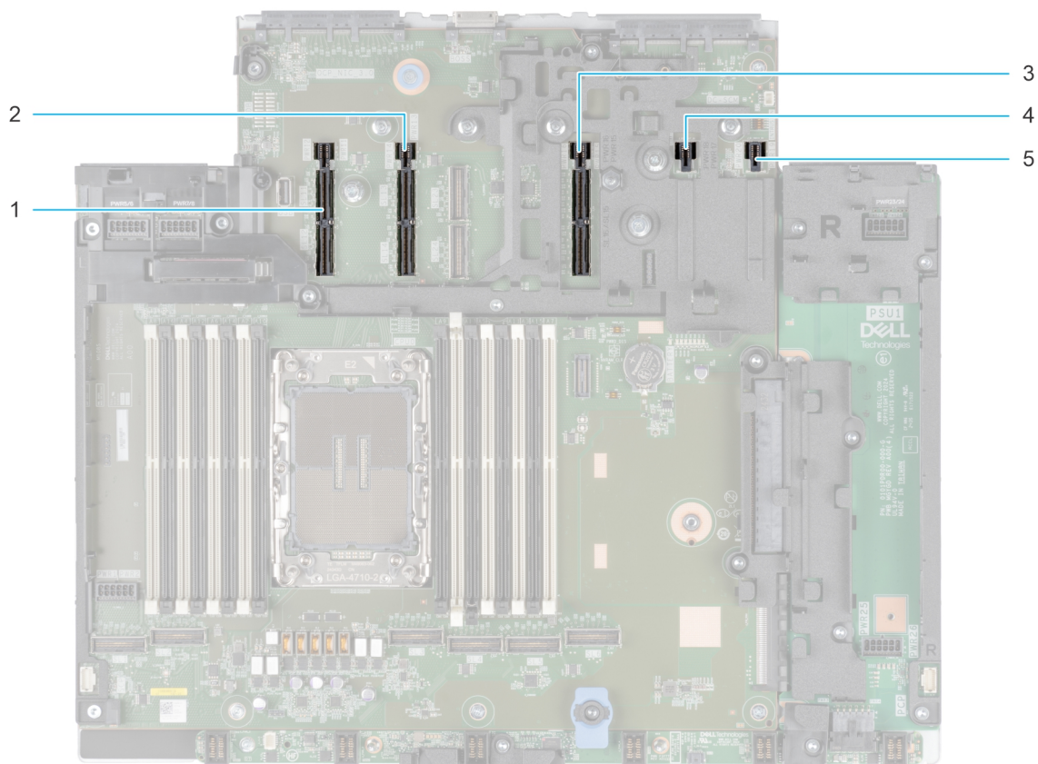
Ilustración 122. Conectores de la ranura de tarjeta elevadora para tarjetas de expansión
