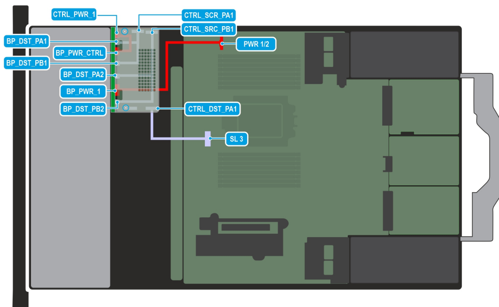
Ilustración 93. Configuración de cables C03-09 8: 8 unidades de 2,5 pulgadas (G4 NVMe RAID)
