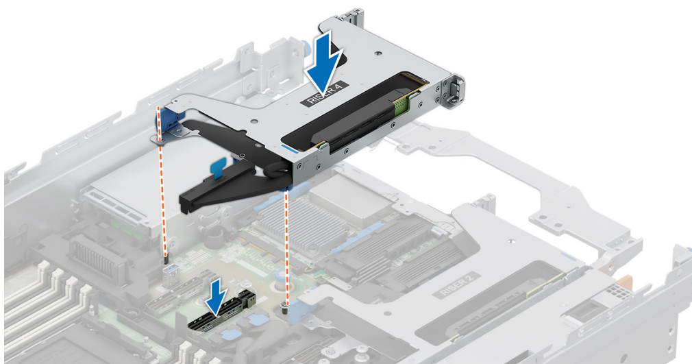
Ilustración 151. Instalación de la tarjeta elevadora para tarjetas de expansión posterior 4
