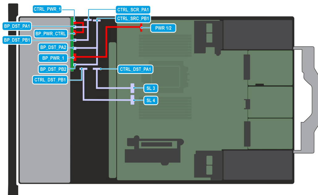
Ilustración 92. Configuración de cables C03-08 7: 8 unidades de 2,5 pulgadas (G4 NVMe RAID)
