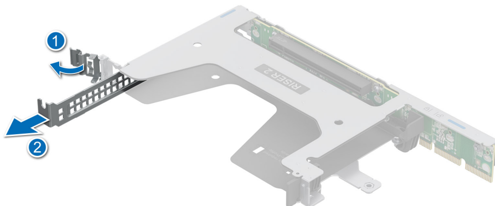
Ilustración 168. Extracción del soporte de relleno
