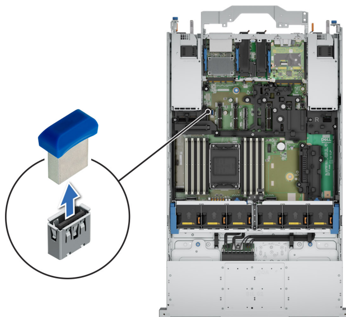
Ilustración 245. Extracción de la tarjeta USB interna
