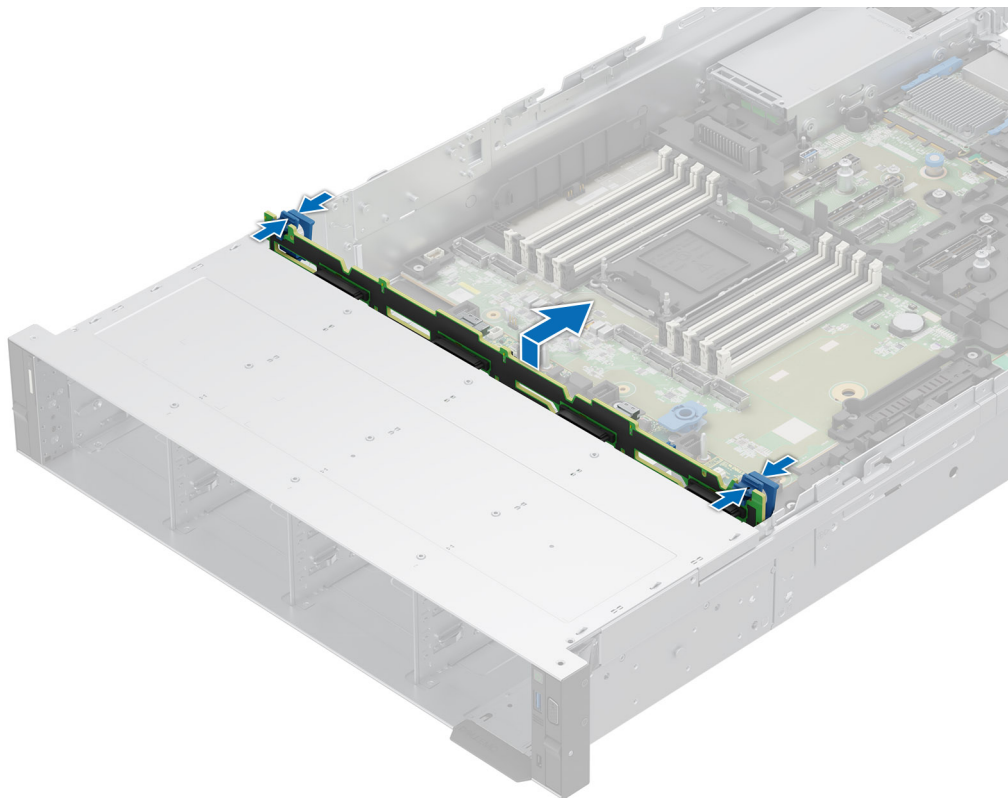
Ilustración 71. Extracción del módulo del backplane de unidades de 3,5 pulgadas
