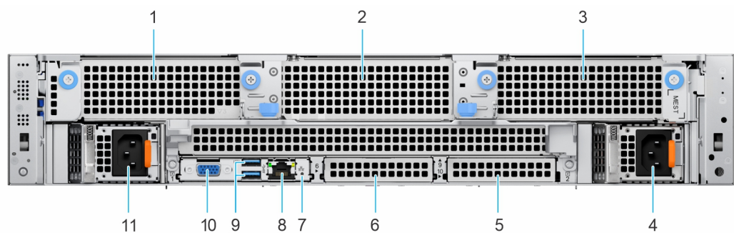
Ilustración 10. Vista posterior del sistema con configuración de I/O frontal
