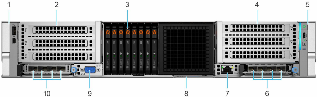
Ilustración 2. Vista frontal de un sistema de 8 unidades EDSFF E3.S NVMe (pasillo frío)
