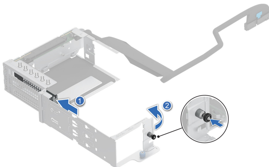
Ilustración 142. Instalación del soporte de relleno
