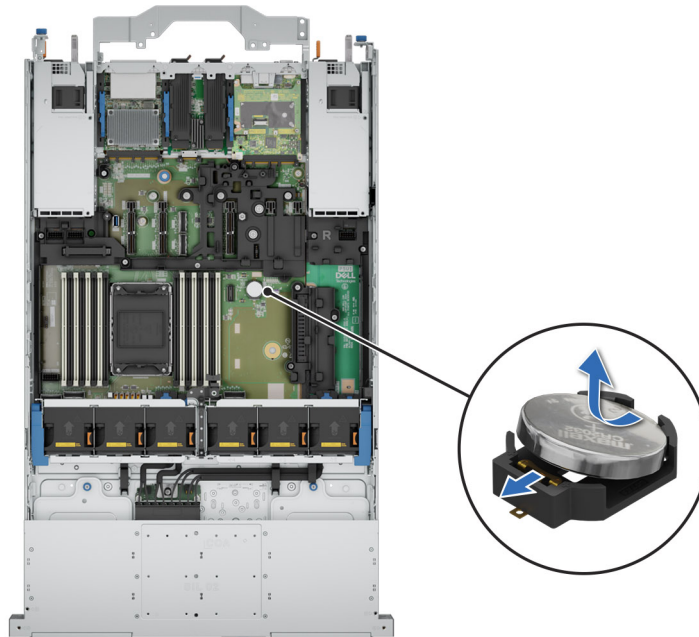
Ilustración 247. Extracción de la batería del sistema
