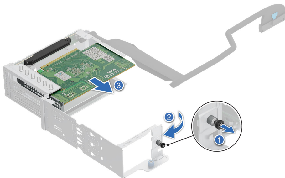
Ilustración 140. Extracción de una tarjeta de expansión de FH de la tarjeta elevadora para tarjetas de expansión frontal
