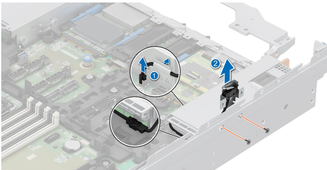
Ilustración 249. Extracción del módulo del switch de intrusión
