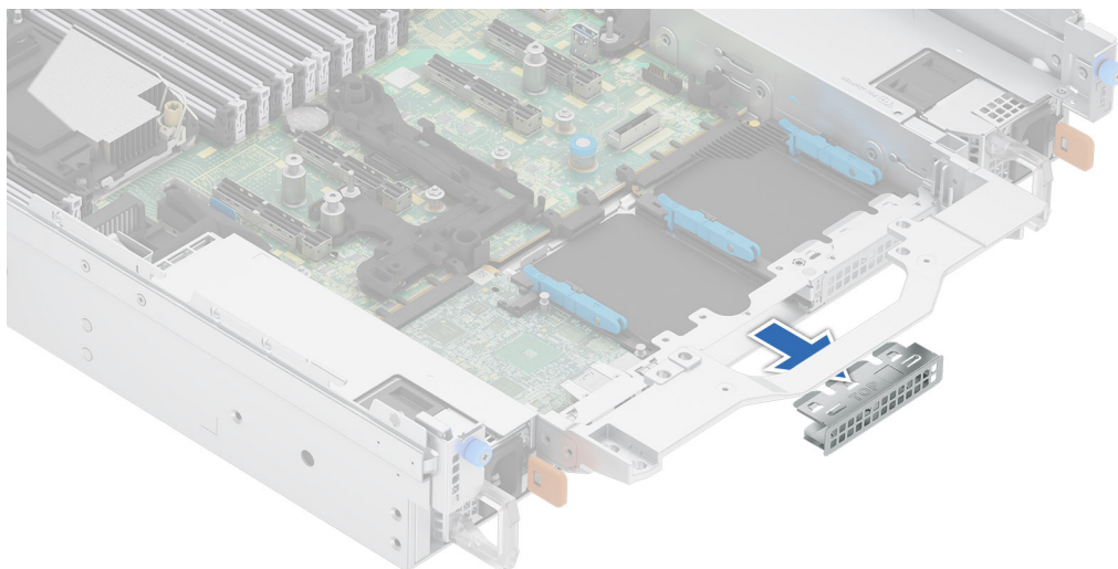
Ilustración 204. Extracción del soporte de relleno
