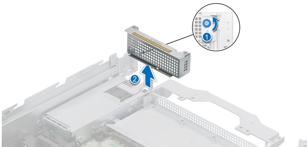
Ilustración 176. Extracción de la tarjeta elevadora para tarjetas de expansión posterior de relleno 5
