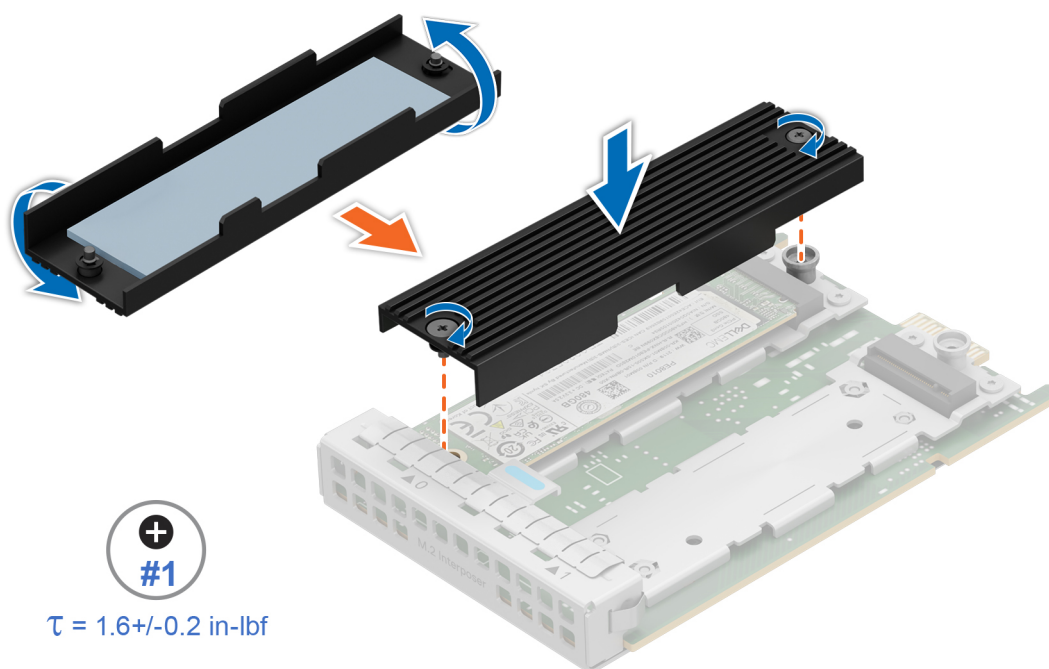
Ilustración 201. Instalación de la cubierta superior
