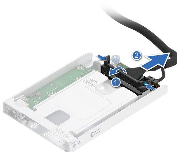
Ilustración 229. Extracción de un cable de NIC de OCP
