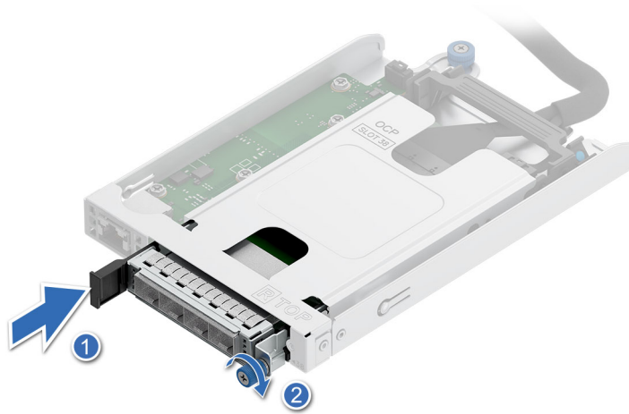
Ilustración 235. Instalación de la bandeja de NIC de OCP en la tarjeta elevadora
