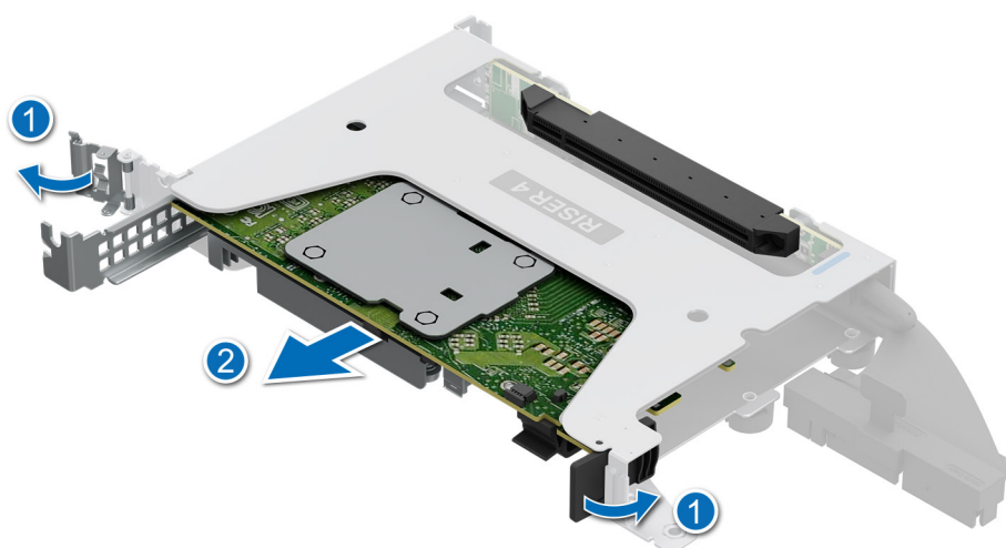
Ilustración 162. Extracción de la tarjeta de expansión de la tarjeta elevadora 4
