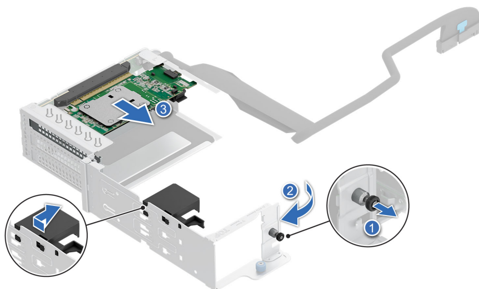
Ilustración 141. Extracción de una tarjeta de expansión de LP de la tarjeta elevadora para tarjetas de expansión frontal
