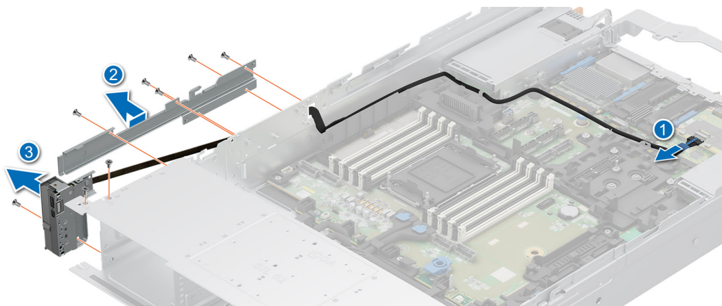
Ilustración 263. Extracción del panel de control izquierdo de KVM
