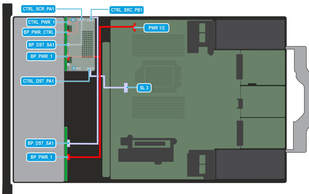
Ilustración 88. Configuración de cables C02-02 3: 16 unidades de 2,5 pulgadas (SAS4/SATA)
