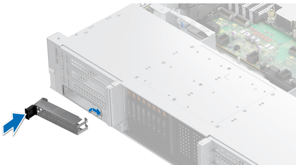
Ilustración 219. Instalación de un soporte de relleno para la controladora BOSS-N1 DC-MHS
