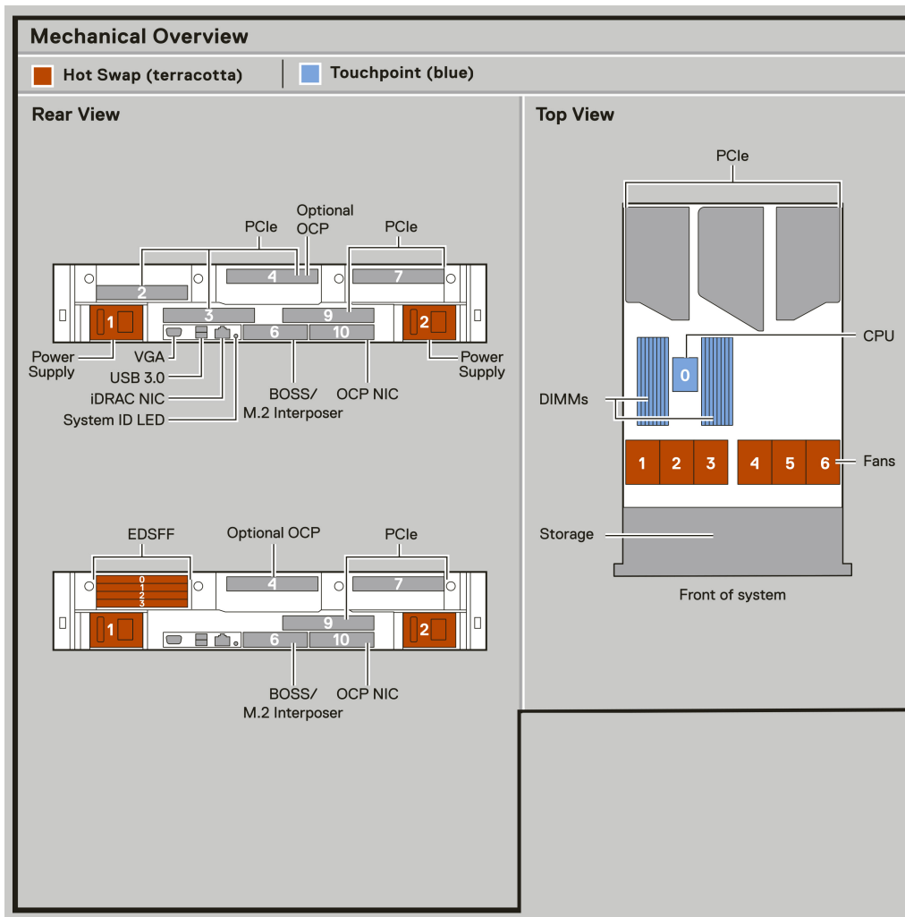
Ilustración 16. Descripción general de los aspectos mecánicos
