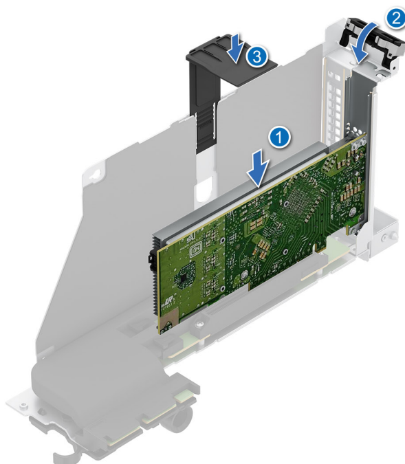
Ilustración 171. Instalación de una tarjeta de expansión en la tarjeta elevadora
