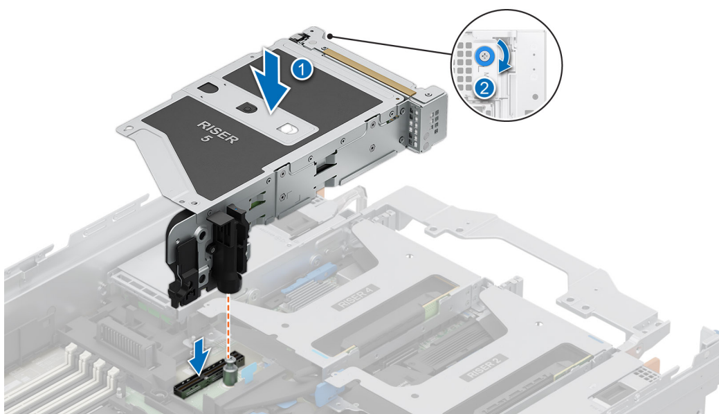
Ilustración 153. Instalación de la tarjeta elevadora para tarjetas de expansión posterior 5
