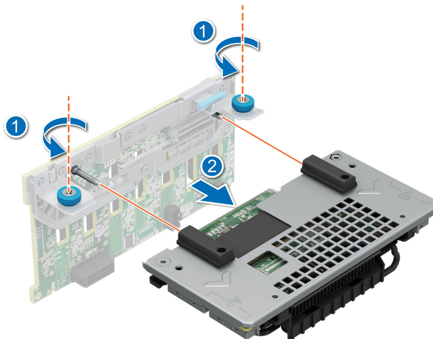
Ilustración 120. Extracción del módulo de fPERC
