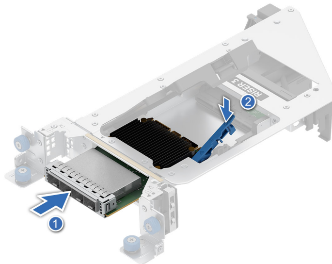
Ilustración 172. Instalación de una tarjeta NIC de OCP en la tarjeta elevadora 3
