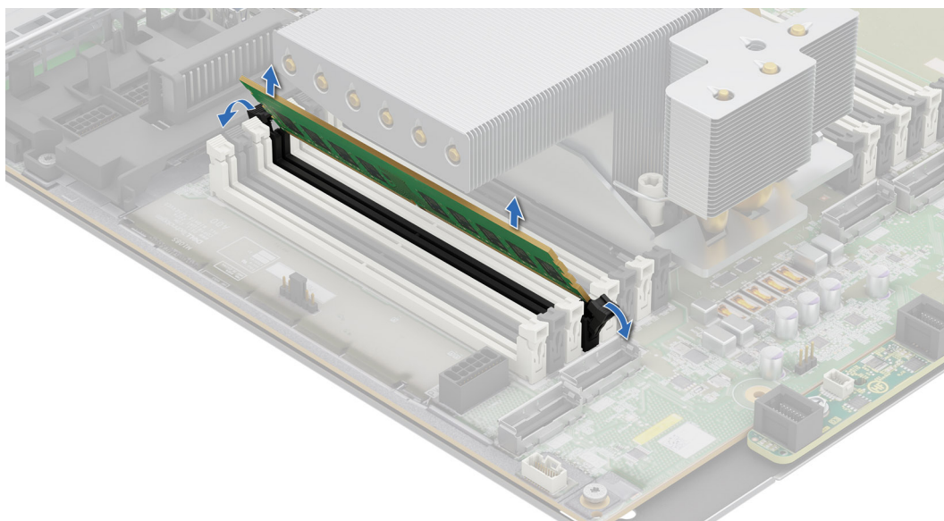
Ilustración 106. Extracción de un módulo de memoria debajo del disipador de calor con aspas
