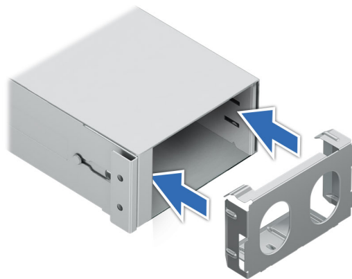
Ilustración 254. Instalación de una fuente de alimentación de relleno
