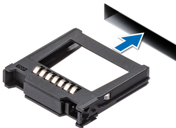
Ilustración 53. Instalación de un disco duro de relleno de 2,5 pulgadas
