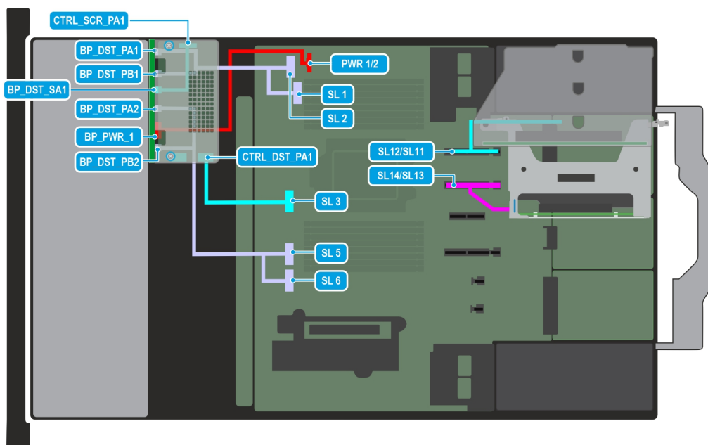
Ilustración 95. C03-012 Configuración de cable 10: 8 x 2,5 pulgadas (universal)
