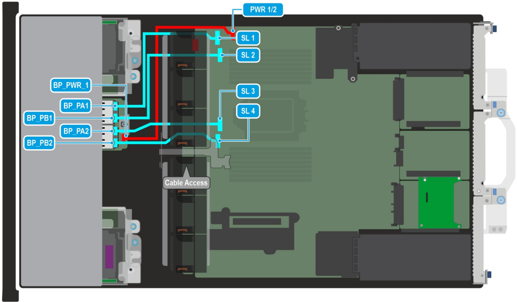
Ilustración 86. Configuración de cables C01-02 1: 8 EDSFF E3.S (NVMe de conexión directa G5x4): pasillo frío
