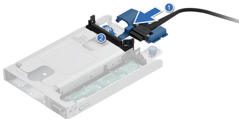
Ilustración 222. Instalación de un cable BOSS-N1 DC-MHS
