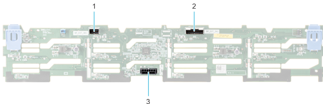
Ilustración 66. Backplane de 12 unidades de 3,5 pulgadas
