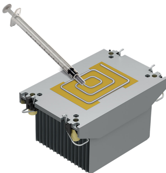
Ilustración 115. Aplicación de la grasa térmica
