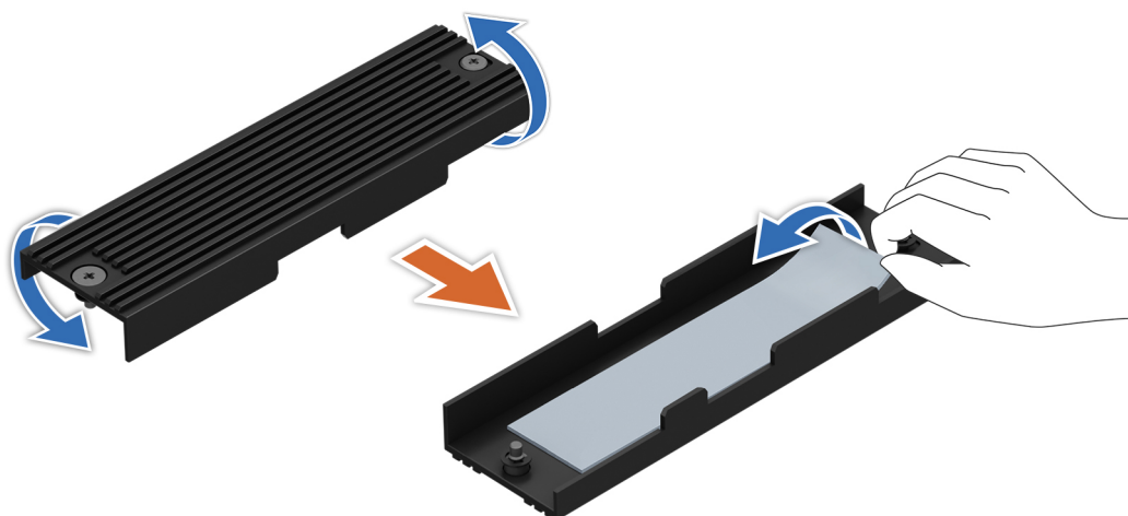
Ilustración 192. Extracción de la almohadilla térmica de la cubierta superior
