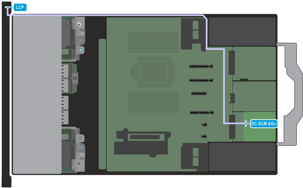
Ilustración 78. Panel de control izquierdo: secundario (LCP) y placa secundaria DC-SCM
