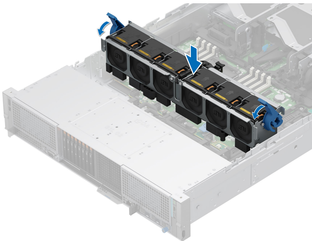
Ilustración 41. Instalación del ensamblaje de la canastilla para el ventilador de enfriamiento
