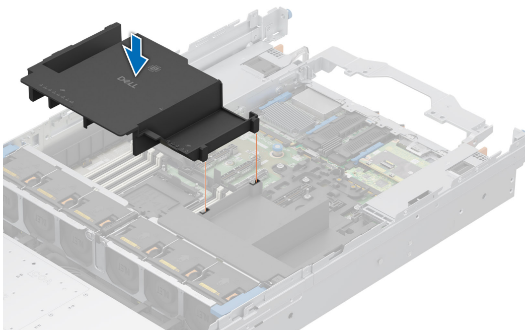
Ilustración 37. Instalación de la cubierta para flujo de aire izquierda
