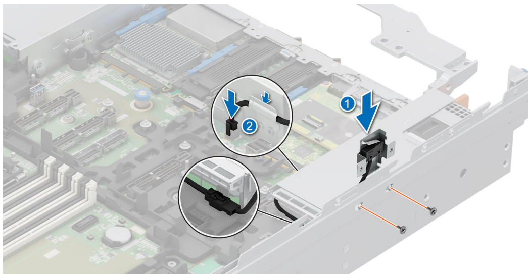
Ilustración 250. Instalación del módulo del switch de intrusión
