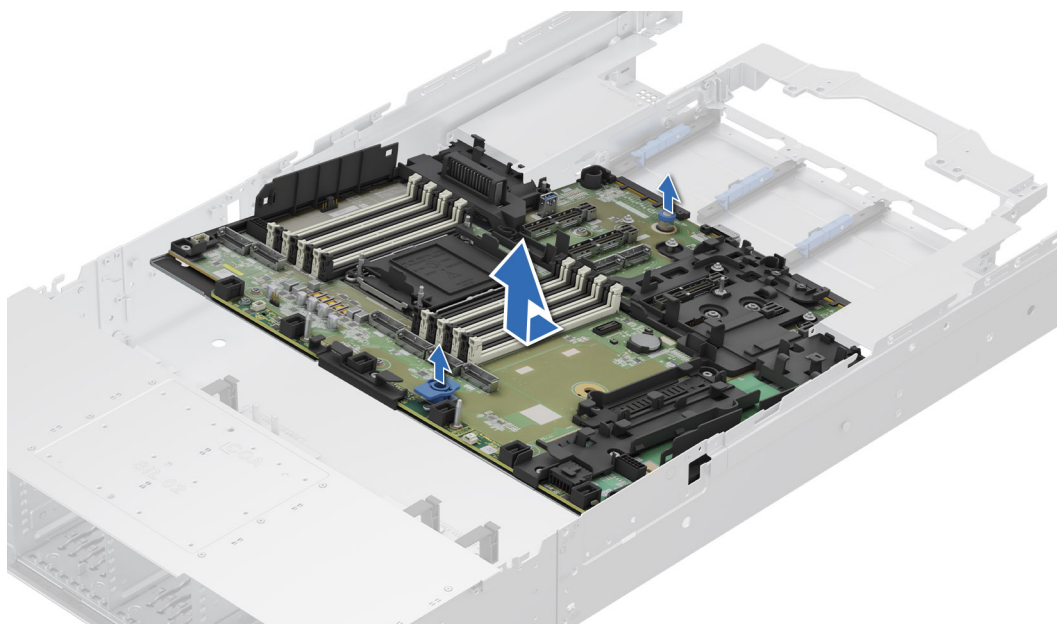
Ilustración 259. Extracción de la placa HPM
