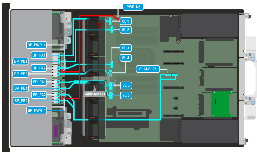
Ilustración 100. C06-01 Configuración de cable 14: 16 EDSFF E3. S (conexión directa NVMe G5x4)
