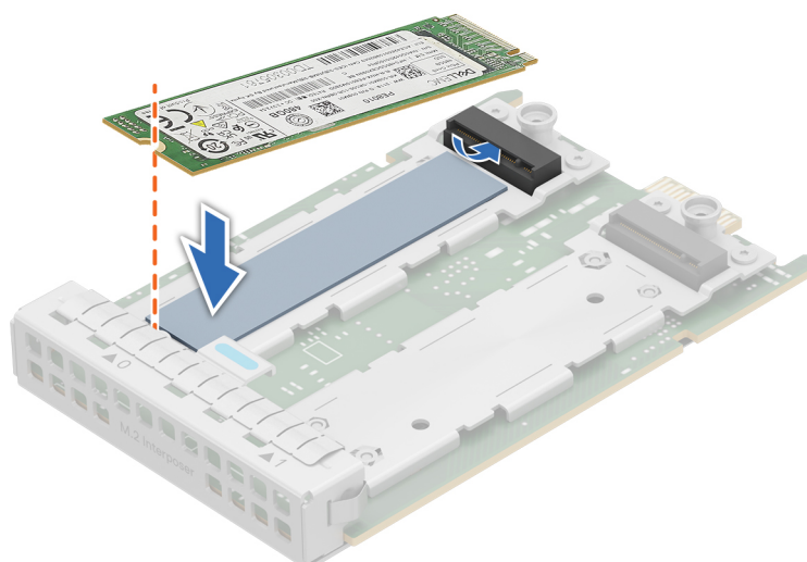
Ilustración 197. Instalación del módulo de SSD NVMe M.2 nuevo
