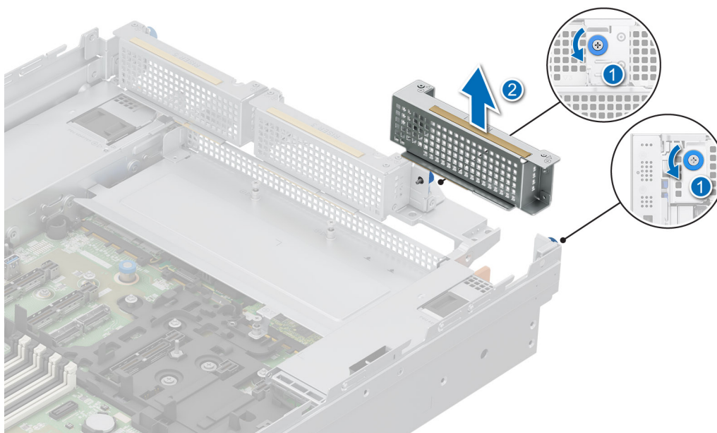
Ilustración 174. Extracción de la tarjeta elevadora para tarjetas de expansión posterior de relleno 1
