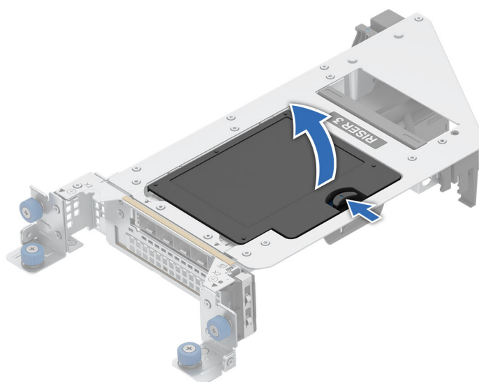
Ilustración 158. Extracción de una cubierta de NIC de OCP de la tarjeta elevadora 3
