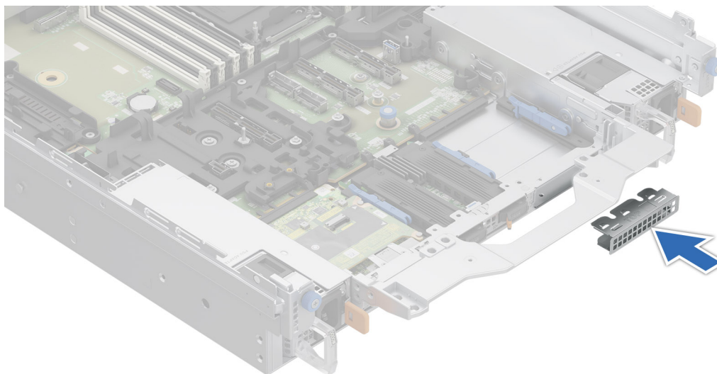
Ilustración 237. Instalación del soporte de relleno
