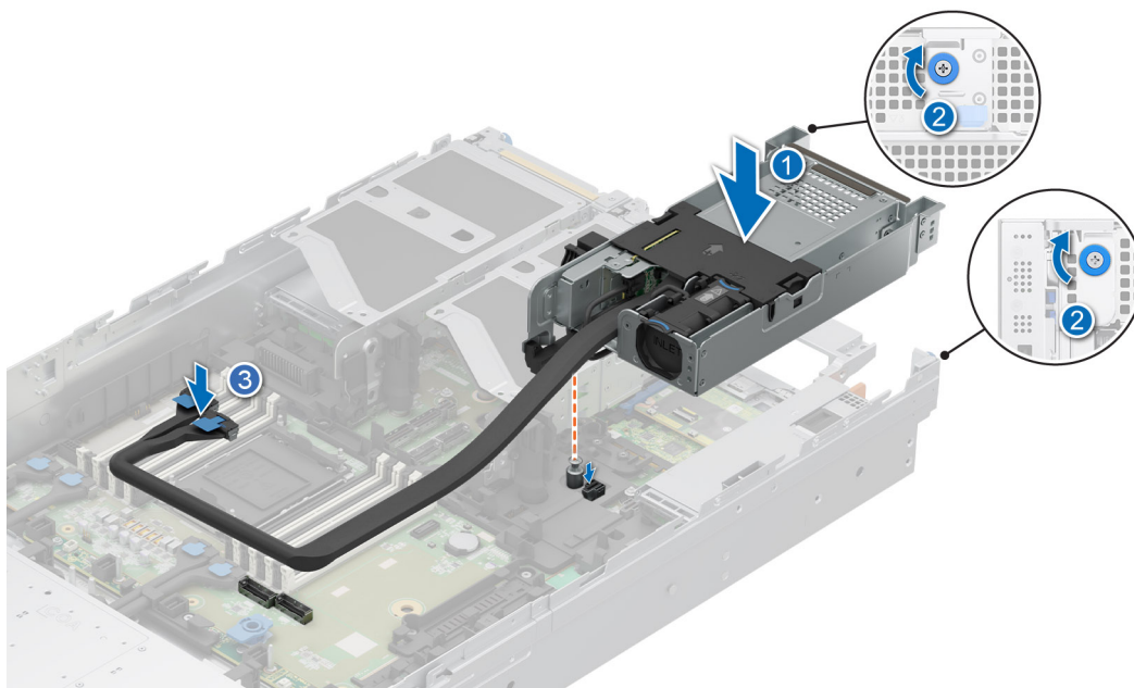
Ilustración 65. Instalación del módulo EDSFF E3.S posterior
