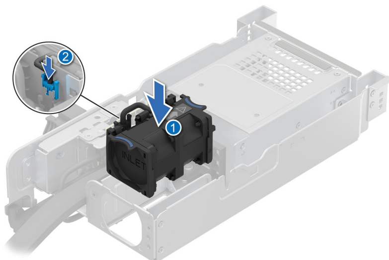
Ilustración 43. Instale el ventilador de enfriamiento del módulo E3.S posterior
