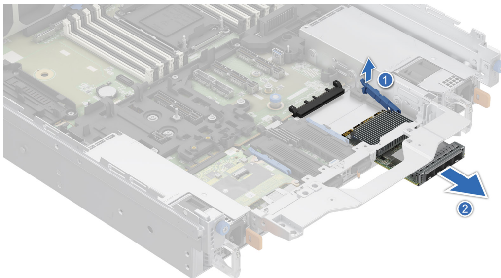
Ilustración 236. Extracción de la tarjeta NIC de OCP posterior
