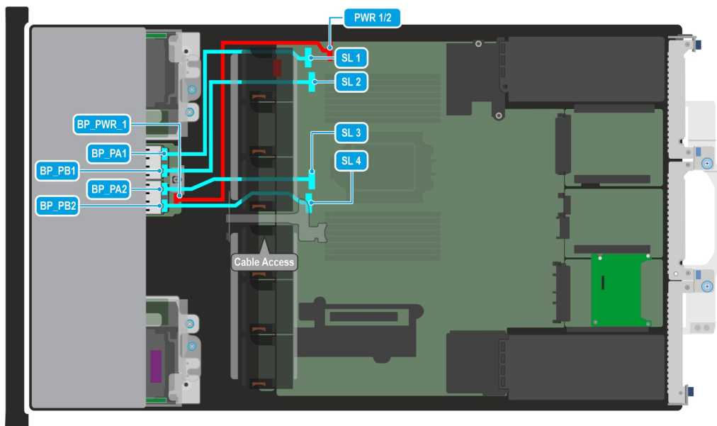
Ilustración 85. Configuración de cables C01-01 0: 8 EDSFF E3.S (NVMe de conexión directa G5x4): pasillo frío
