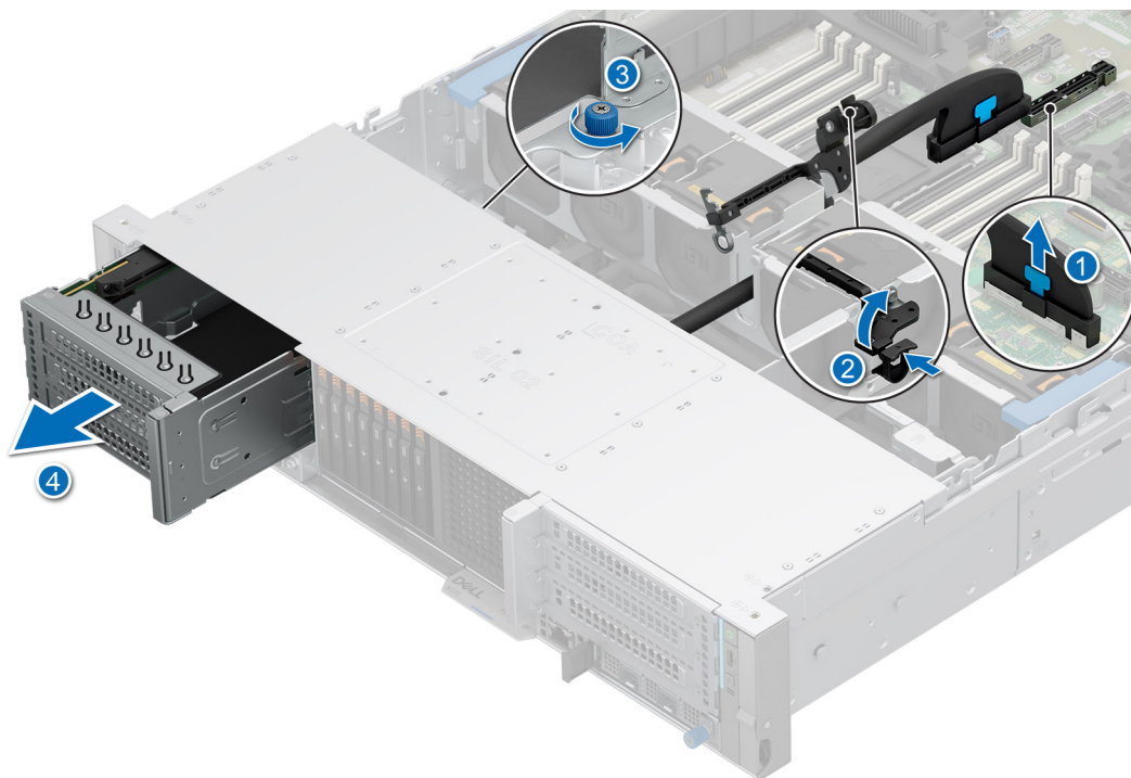
Ilustración 132. Extracción de la tarjeta elevadora para tarjetas de expansión frontal 1
