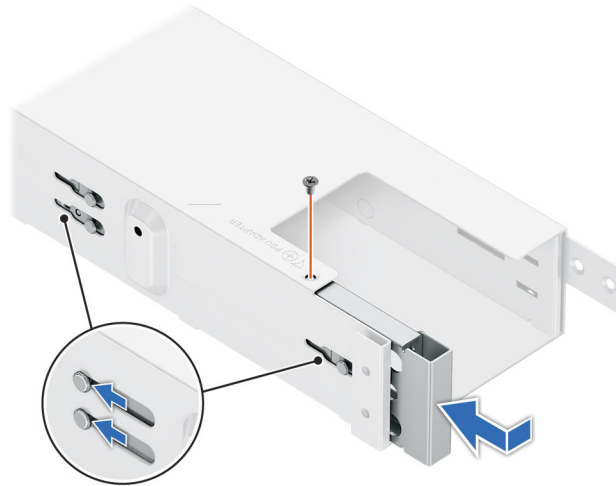
Ilustración 255. Instalación de la PSU de relleno izquierda
