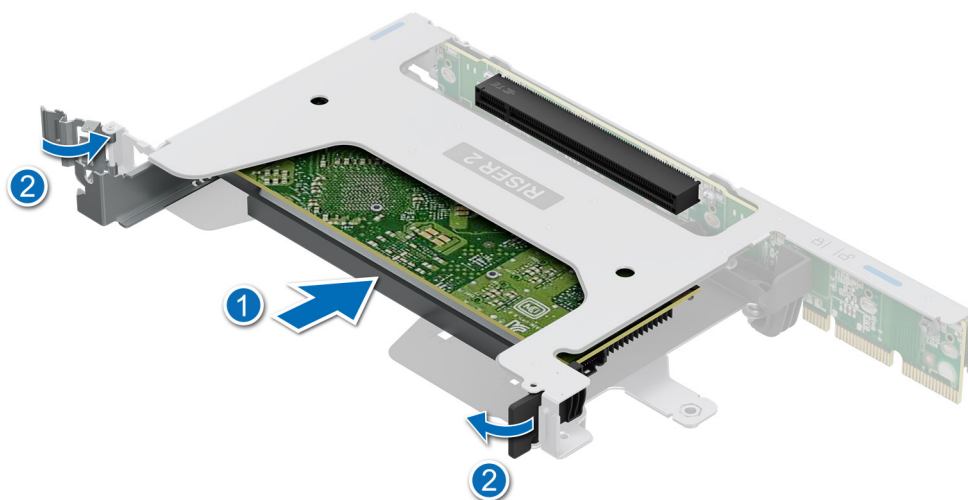
Ilustración 169. Instalación de una tarjeta de expansión en la tarjeta elevadora 2
