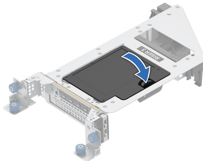
Ilustración 173. Instalación de una cubierta de NIC de OCP en la tarjeta elevadora 3
