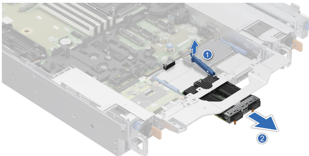
Ilustración 224. Extracción de BOSS-N1 DC-MHS posterior
