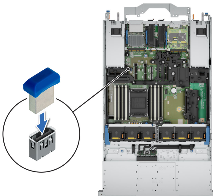
Ilustración 246. Instalación de la tarjeta USB interna
