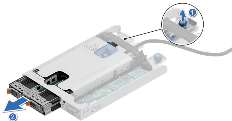
Ilustración 216. Extracción de la bandeja de una controladora BOSS-N1 DC-MHS de la tarjeta elevadora
