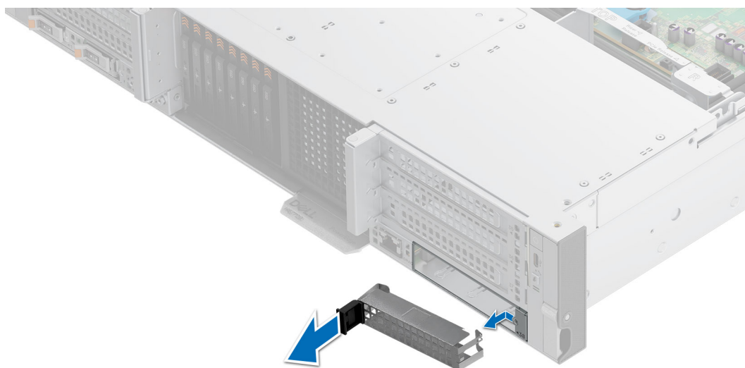
Ilustración 232. Extracción de un soporte de relleno de tarjeta NIC de OCP
