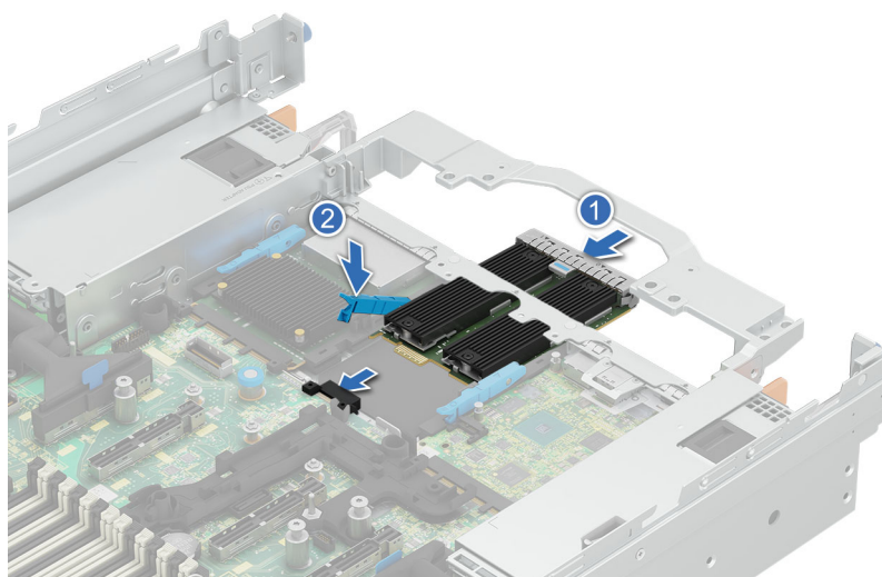
Ilustración 213. Instalación de la placa mediadora de M.2
