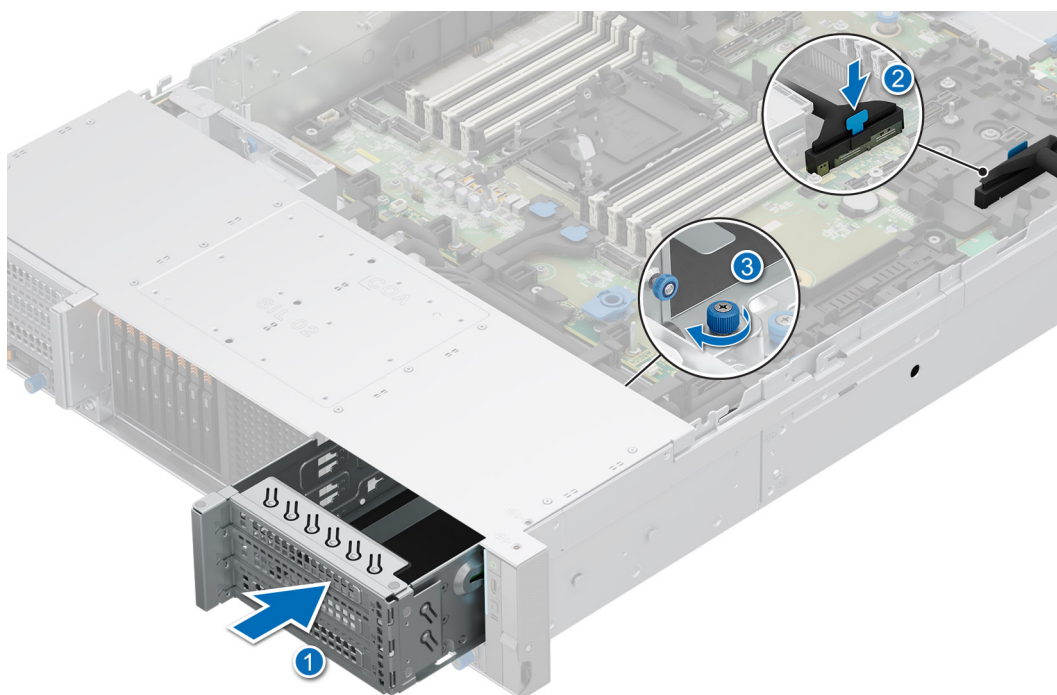
Ilustración 138. Instalación de la tarjeta elevadora para tarjetas de expansión frontal 3
