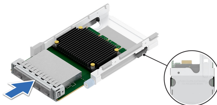
Ilustración 233. Instalación de una tarjeta NIC de OCP en la bandeja de OCP
