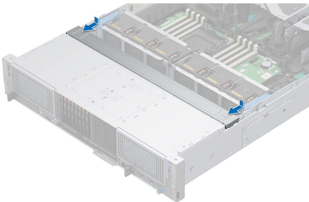
Ilustración 45. Instalación de la cubierta del backplane de la unidad
