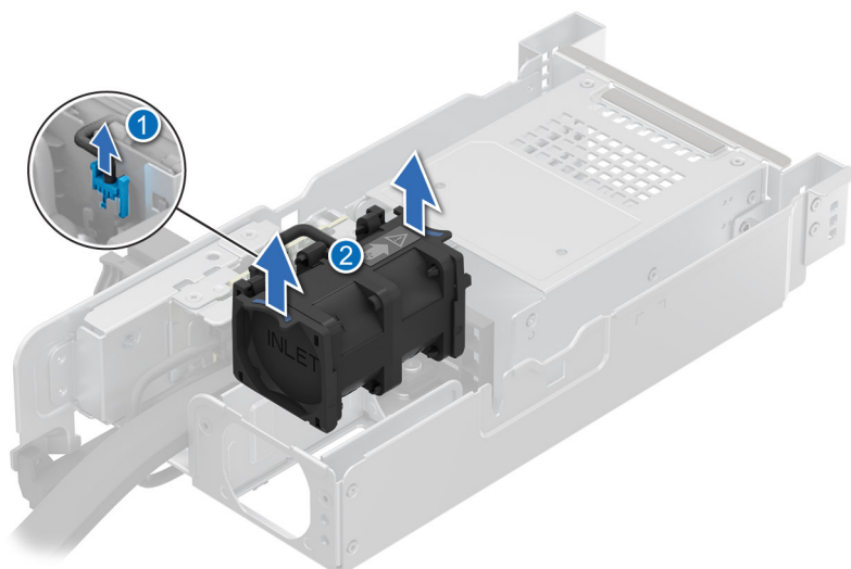
Ilustración 42. Extracción del ventilador de enfriamiento del módulo E3.S posterior
