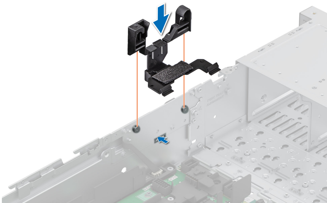
Ilustración 76. Instalación del soporte de pared lateral
