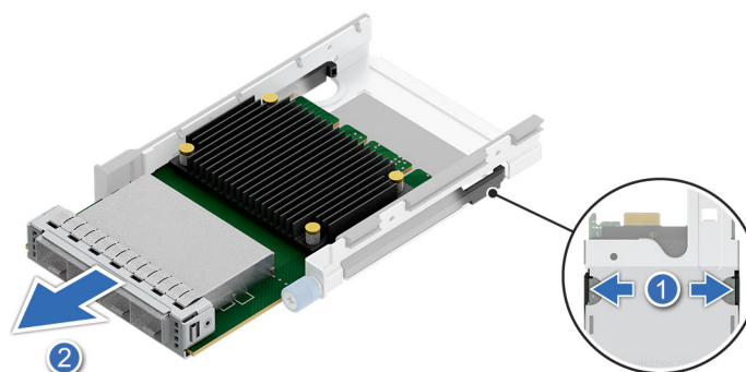
Ilustración 230. Extracción de una tarjeta NIC de OCP de la bandeja de OCP
