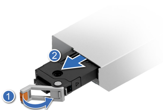
Ilustración 182. Extracción del portaunidades de tarjeta BOSS-N1
