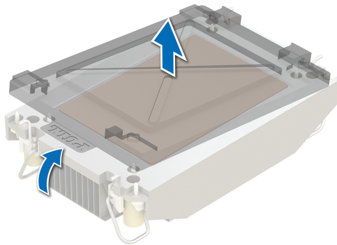
Ilustración 116. Extracción de la cubierta
