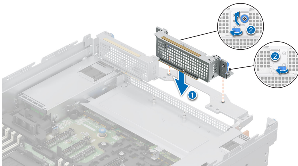
Ilustración 180. Instalación de la tarjeta elevadora para tarjetas de expansión posterior de relleno 3
