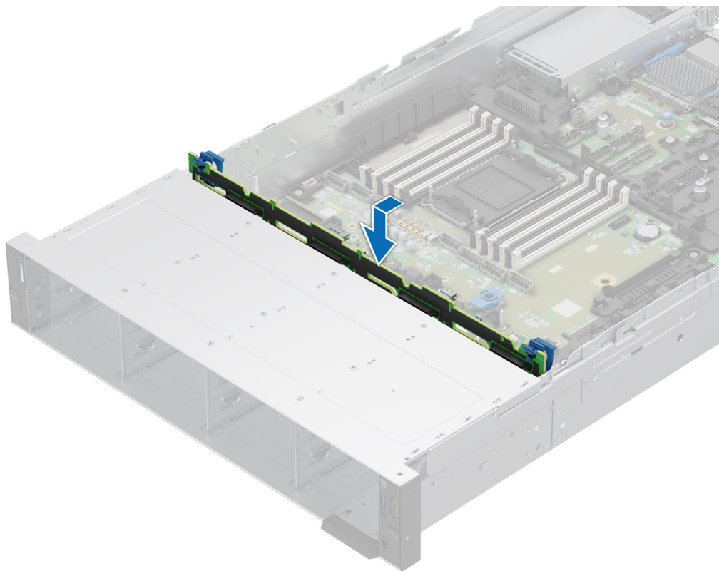
Ilustración 72. Instalación del módulo de backplane para unidades de 3,5 pulgadas
