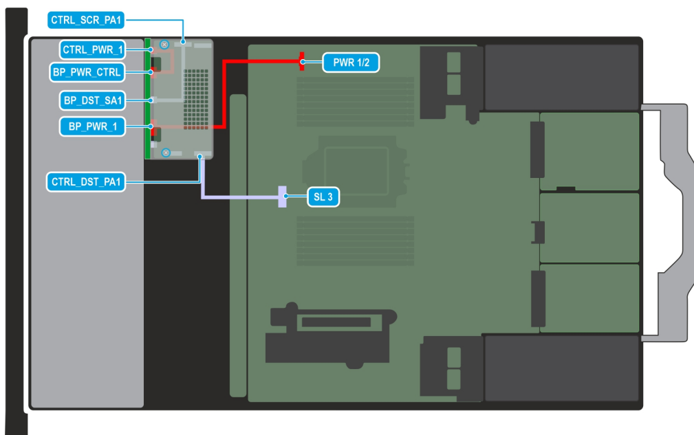
Ilustración 90. Configuración de cables C03-02 5: 8 unidades de 2,5 pulgadas (SAS4/SATA)
