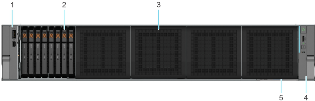
Ilustración 7. Vista frontal de 8 x EDSFF E3. Sistema de unidades S NVMe (pasillo caliente)
