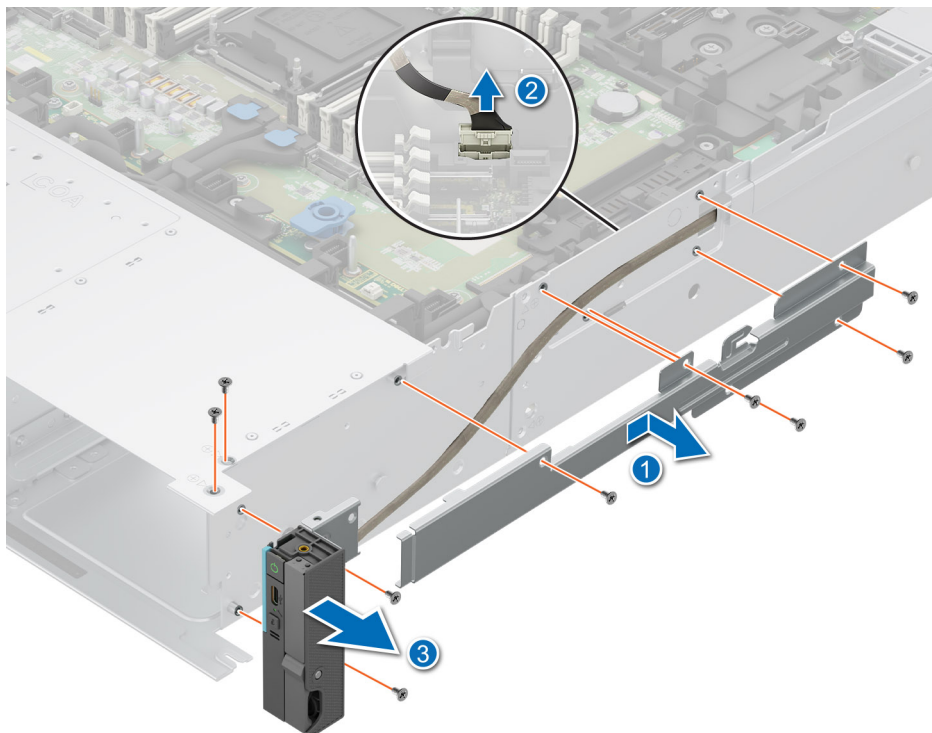
Ilustración 261. Extracción del panel de control derecho: principal
