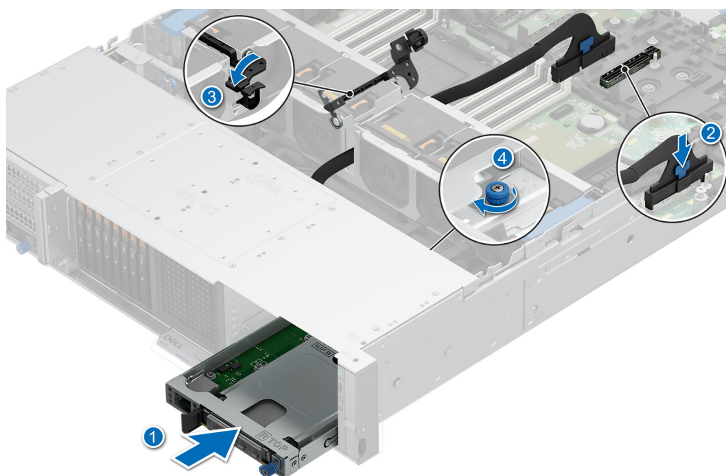
Ilustración 137. Instalación de la tarjeta elevadora para tarjetas de expansión frontal 4
