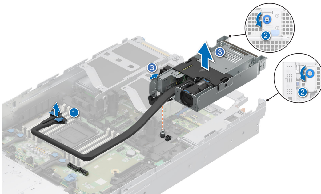
Ilustración 64. Extracción del módulo posterior de 4 EDSFF E3.S
