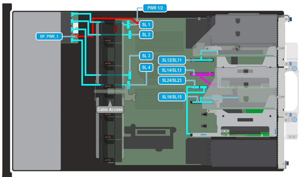
Ilustración 102. C08-01 Configuración de cable 22: 8 EDSFF E3. S (conexión directa NVMe G5x4)
