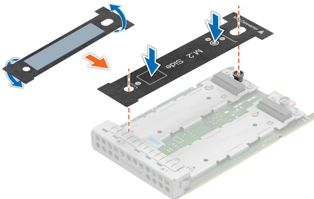
Ilustración 195. Giro e instalación de la nueva almohadilla térmica en la placa
