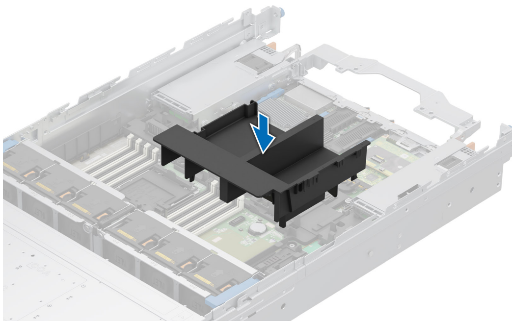
Ilustración 36. Instalación de la cubierta para flujo de aire derecha
