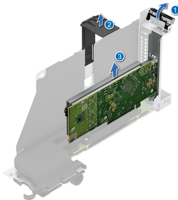
Ilustración 156. Extracción de una tarjeta de expansión de la tarjeta elevadora para tarjetas de expansión posterior
