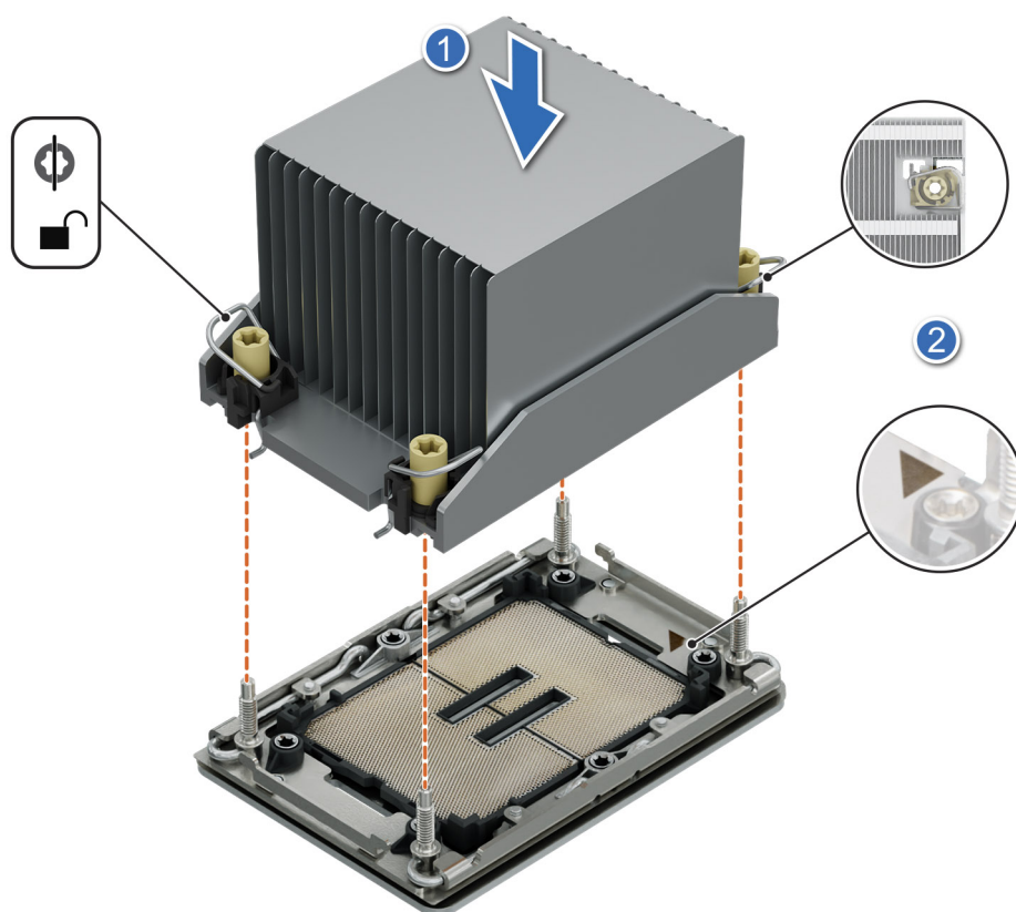
Ilustración 118. Instalación del disipador de calor del procesador
