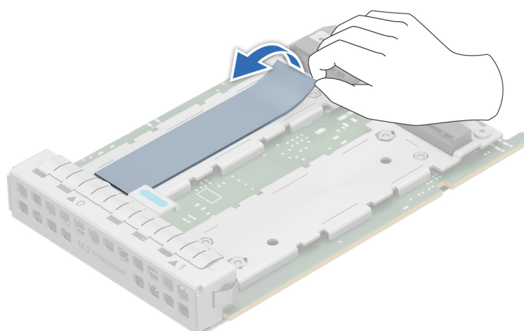
Ilustración 193. Extracción de la almohadilla térmica de la placa de la ranura 0
