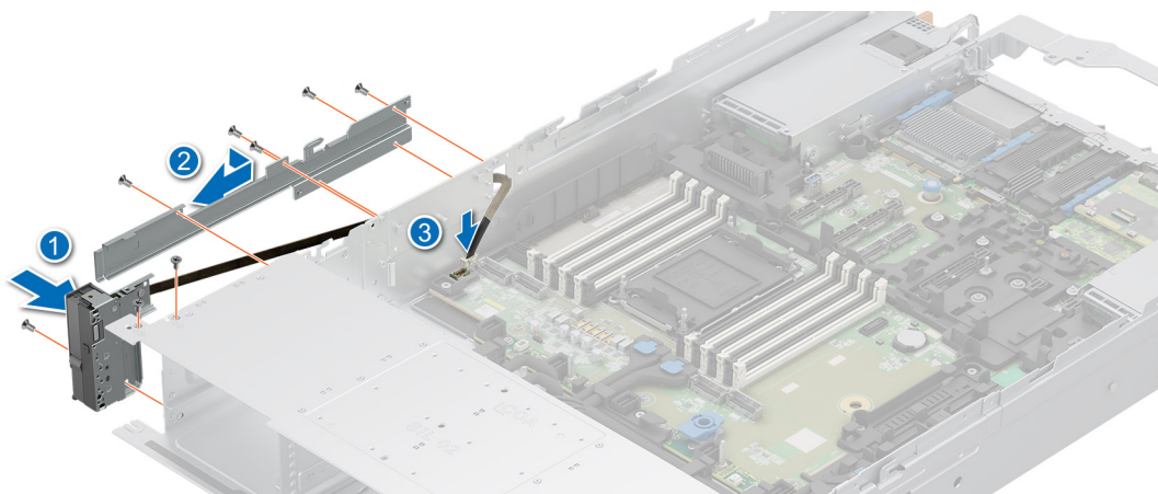
Ilustración 266. Instalación del panel de control izquierdo de Quick Sync
