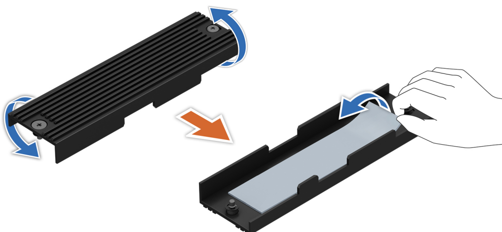
Ilustración 208. Giro de la cubierta superior y extracción de la almohadilla térmica de la cubierta superior
