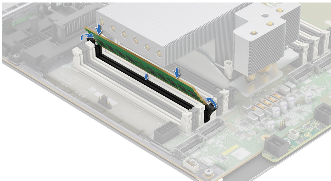
Ilustración 108. Instalación de un módulo de memoria debajo del disipador de calor con aspas
