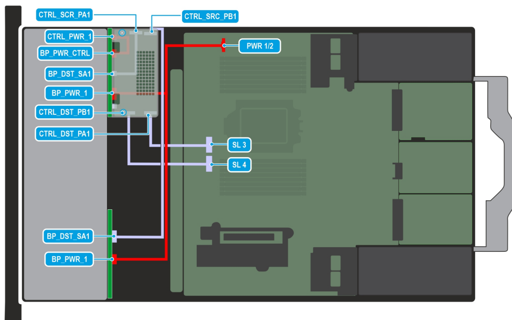
Ilustración 87. Configuración de cables C02-01 2: 16 unidades de 2,5 pulgadas (SAS4/SATA)
