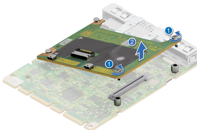
Ilustración 243. Extracción de la placa secundaria
