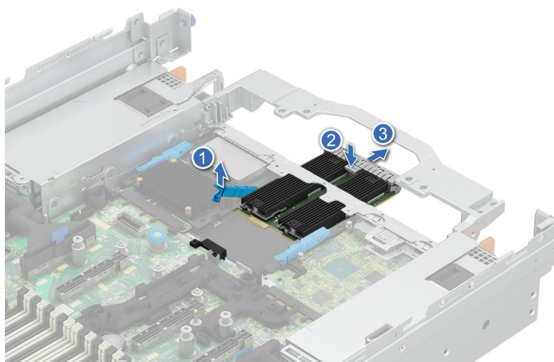
Ilustración 202. Extracción de la placa mediadora de M.2
