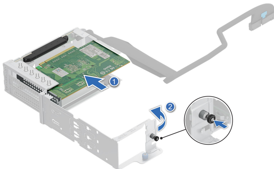
Ilustración 145. Instalación de una tarjeta de expansión de FH en la tarjeta elevadora para tarjetas de expansión frontal
