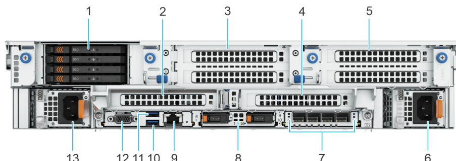
Ilustración 12. Vista posterior del sistema con unidades NVMe EDSFF E3.S posteriores
