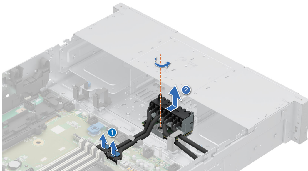
Ilustración 73. Extracción del módulo de backplane EDSFF E3.S
