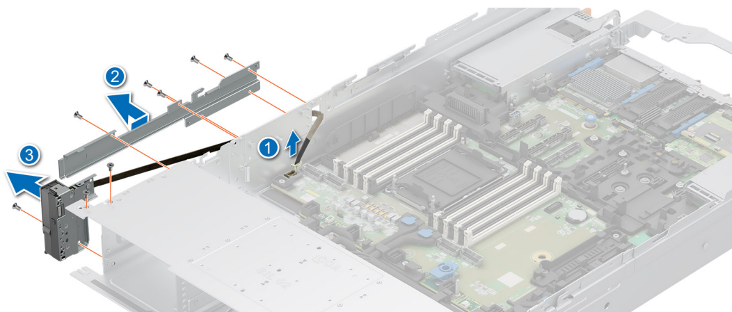
Ilustración 264. Extracción del panel de control izquierdo de Quick Sync
