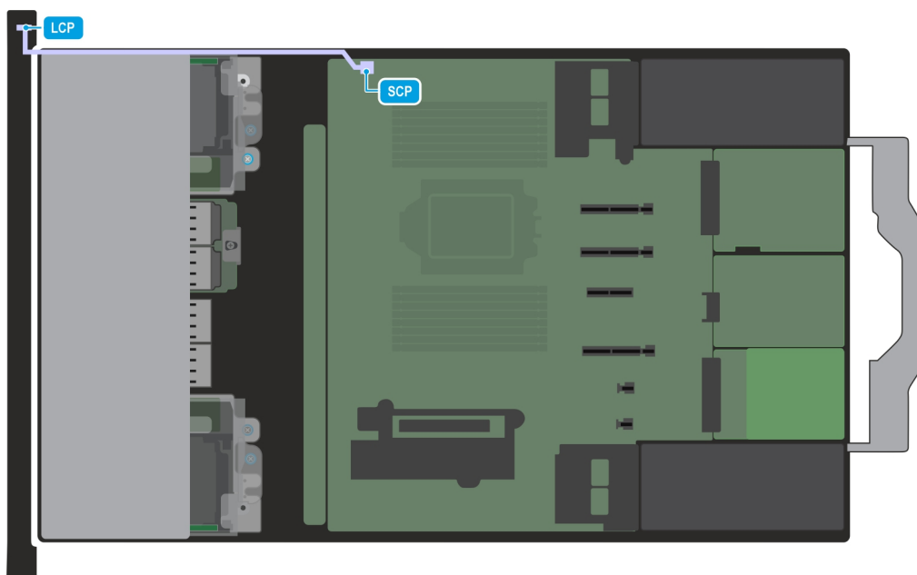
Ilustración 79. Panel de control izquierdo: módulo secundario (LCP) Quick Sync
