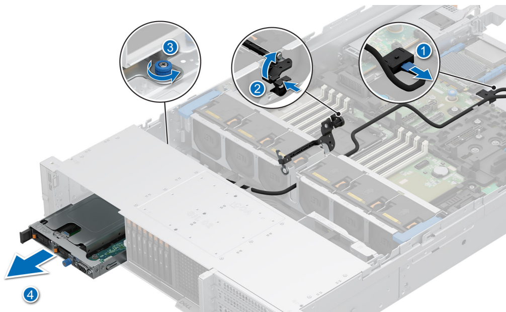
Ilustración 134. Extracción de la tarjeta elevadora para tarjetas de expansión frontal 2
