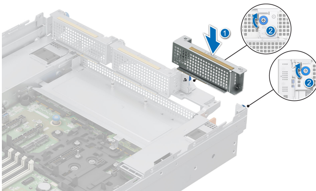
Ilustración 181. Instalación de la tarjeta elevadora para tarjetas de expansión posterior de relleno 1
