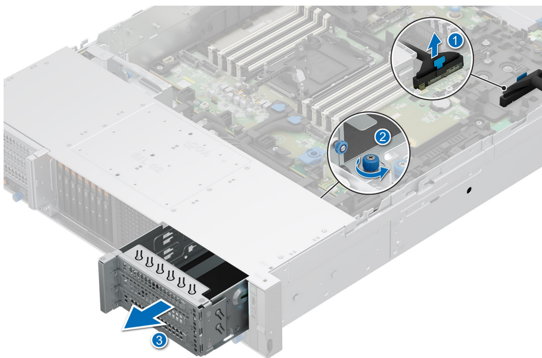
Ilustración 133. Extracción de la tarjeta elevadora para tarjetas de expansión frontal 3
