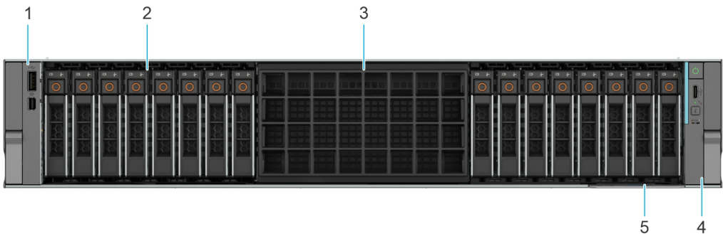
Ilustración 5. Vista frontal de un sistema de 16 unidades de 2,5 pulgadas
