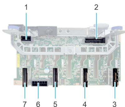
Ilustración 68. Backplane de unidad universal de 8 unidades de 2,5 pulgadas
