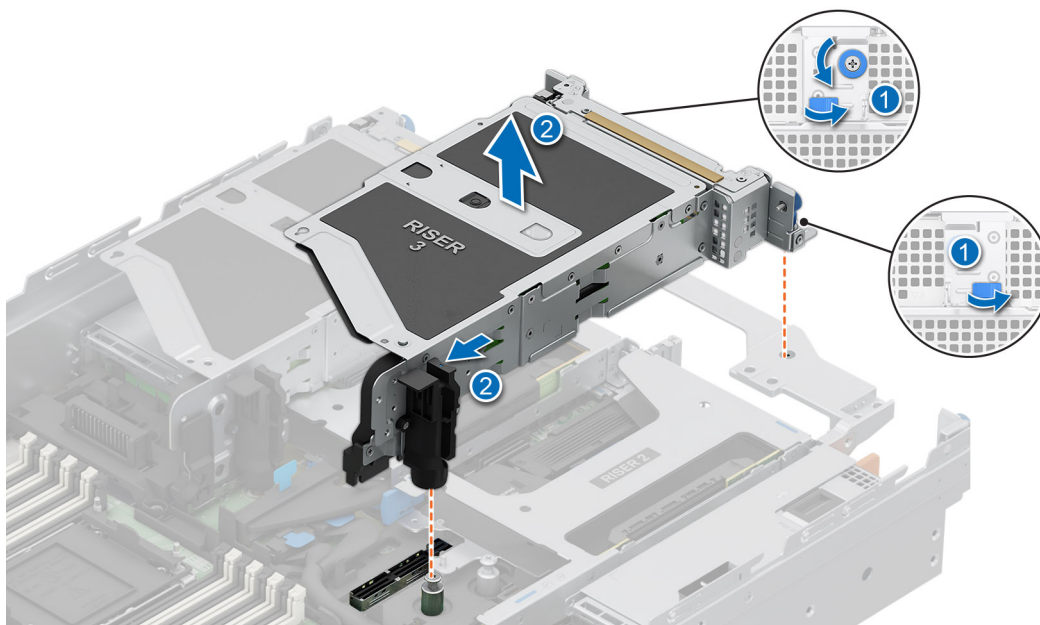
Ilustración 147. Extracción de la tarjeta elevadora para tarjetas de expansión posterior 3
