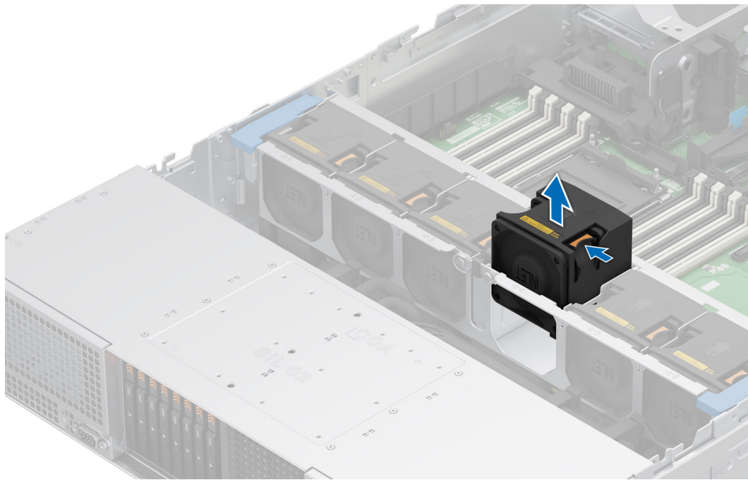
Ilustración 38. Extracción de un ventilador
