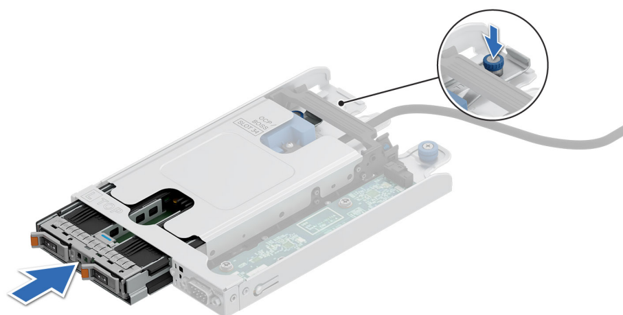
Ilustración 223. Instalación de la bandeja de una controladora BOSS-N1 DC-MHS en la tarjeta elevadora
