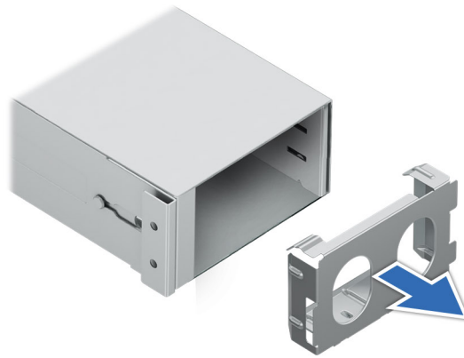
Ilustración 253. Extracción de una fuente de alimentación de relleno
