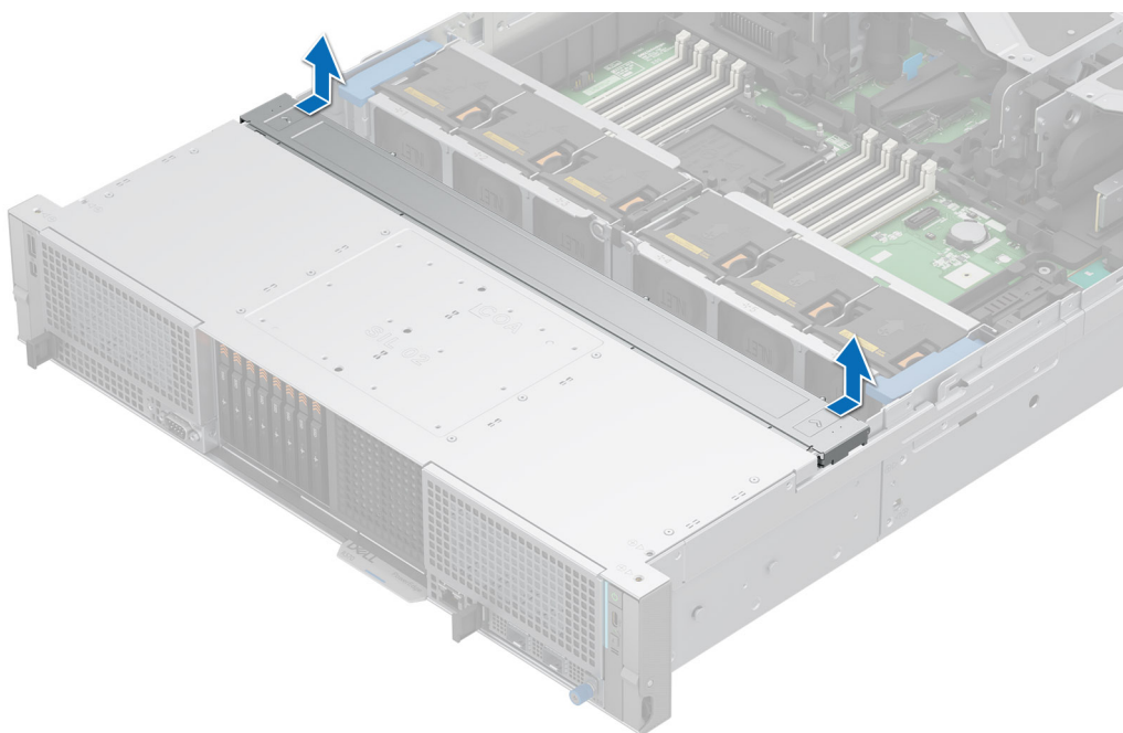
Ilustración 44. Extracción de la cubierta del backplane de la unidad
