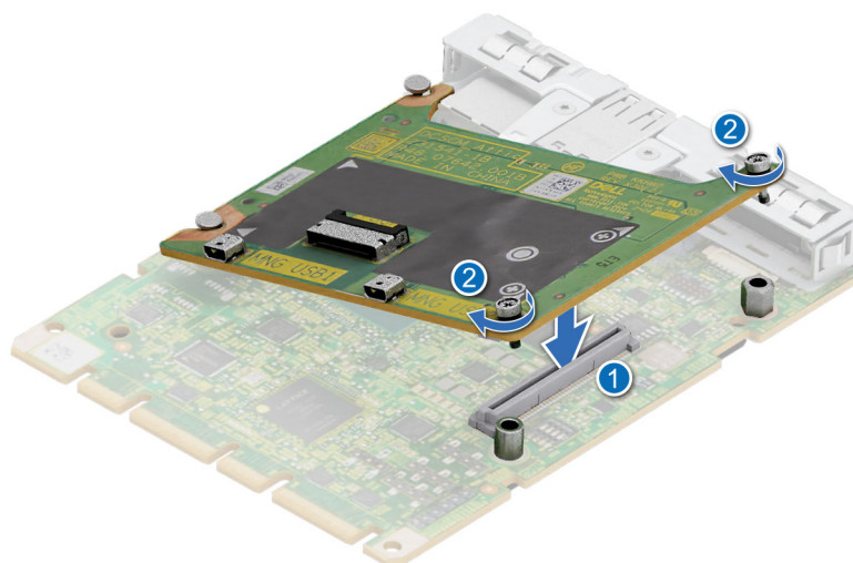
Ilustración 244. Instalación de la placa secundaria
