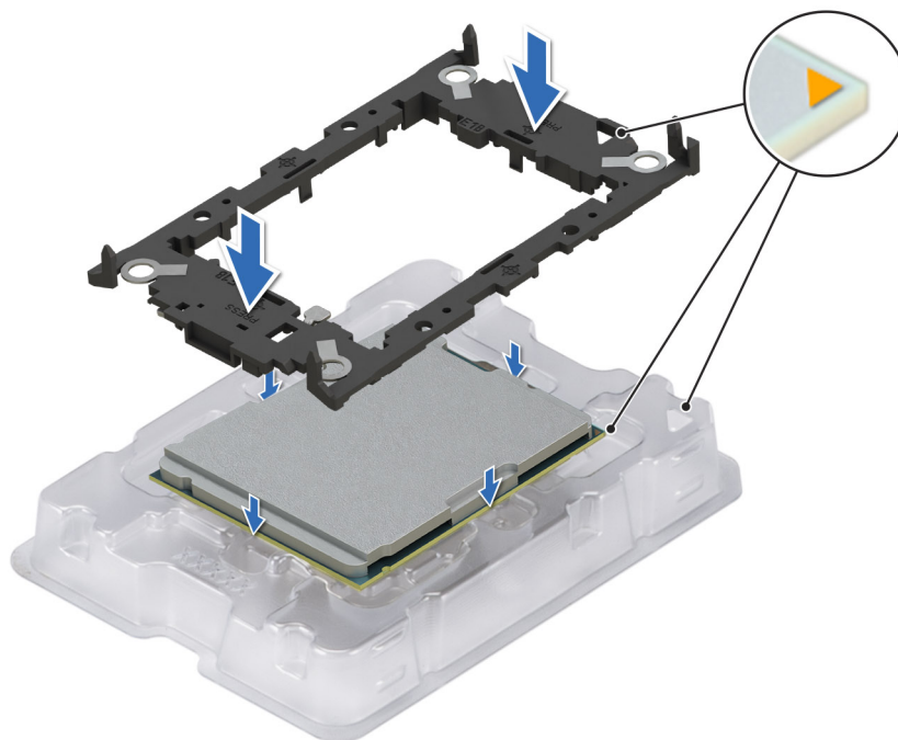
Ilustración 113. Instalación del gancho de retención
