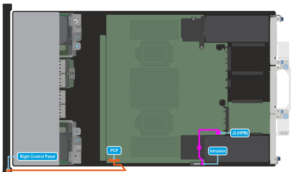
Ilustración 77. Panel de control derecho: principal (RCP) e intrusión
