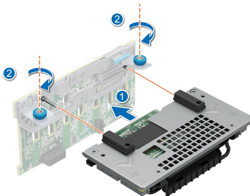
Ilustración 121. Instalación del módulo de fPERC
