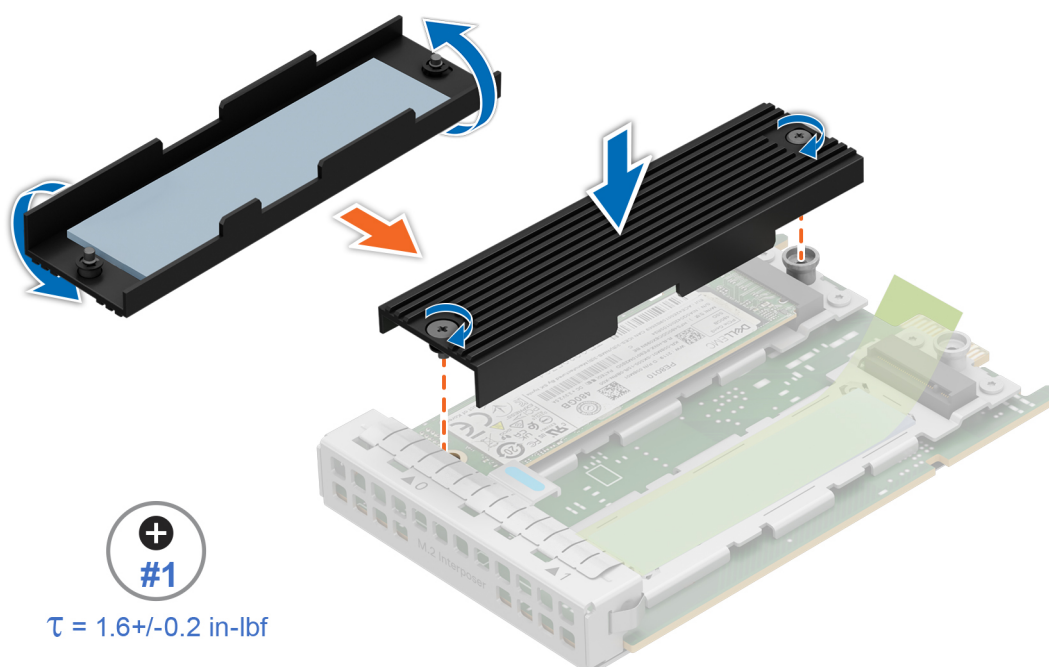
Ilustración 212. Instalación de la cubierta superior en la placa mediadora de M.2
