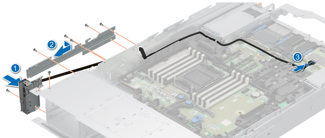
Ilustración 265. Instalación del panel de control izquierdo de KVM
