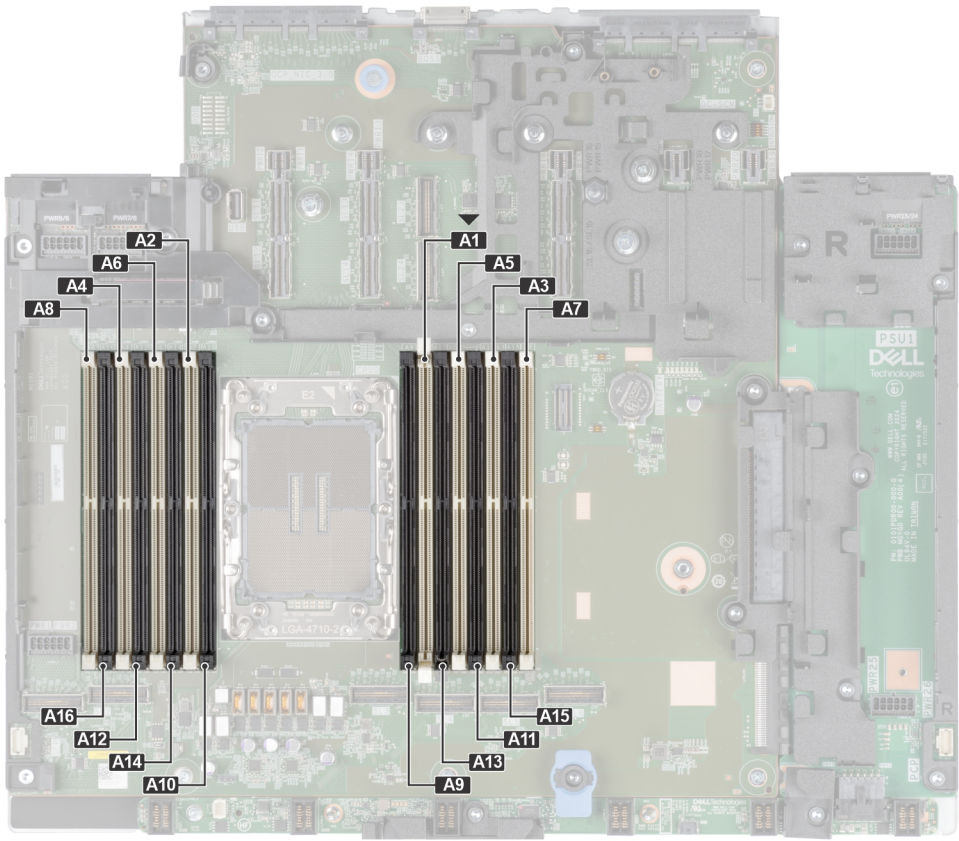
Ilustración 104. Canales de la memoria
