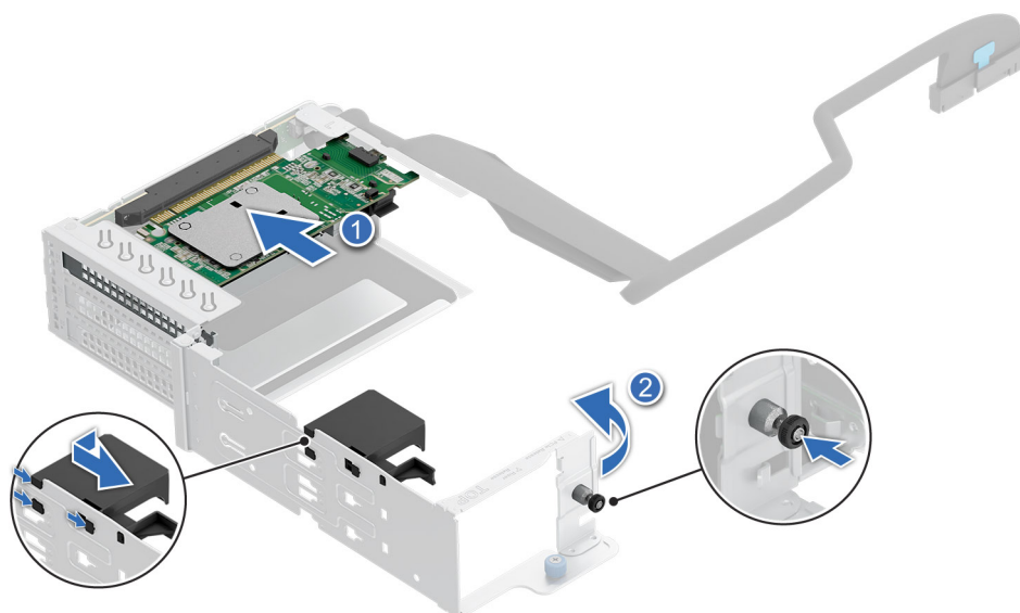
Ilustración 144. Instalación de una tarjeta de expansión de LP en la tarjeta elevadora para tarjetas de expansión frontal
