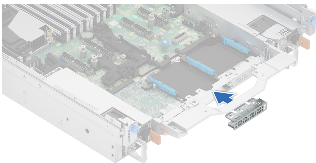
Ilustración 203. Instalación del soporte de relleno
