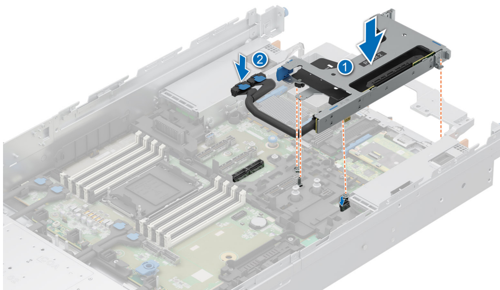
Ilustración 152. Instalación de la tarjeta elevadora para tarjetas de expansión posterior 2
