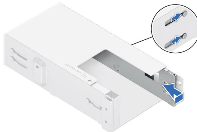
Ilustración 258. Instalación de la PSU de relleno derecha
