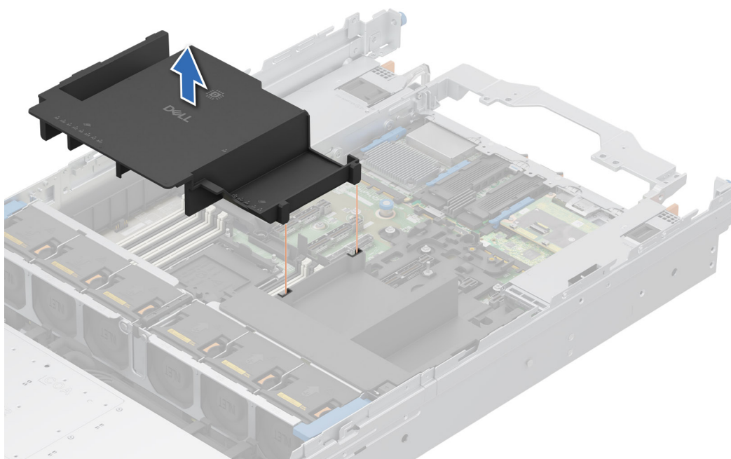
Ilustración 34. Extracción de la cubierta para flujo de aire izquierda
