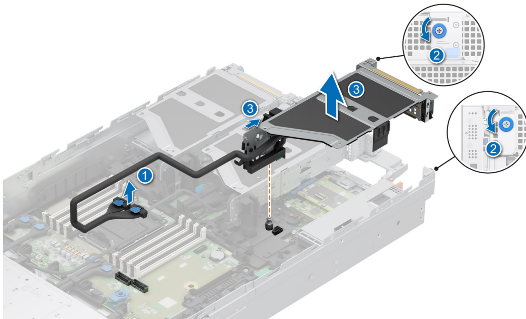
Ilustración 146. Extracción de la tarjeta elevadora para tarjetas de expansión posterior 1
