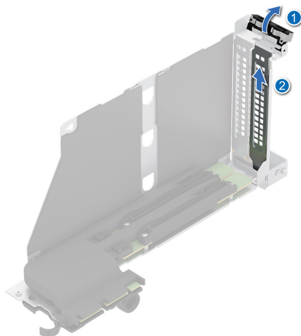
Ilustración 170. Extracción del soporte de relleno
