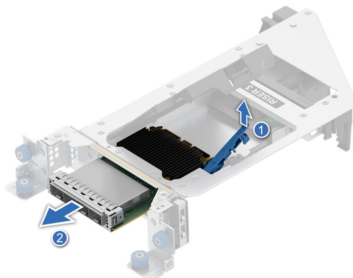
Ilustración 159. Extracción de una tarjeta NIC de OCP de la tarjeta elevadora 3
