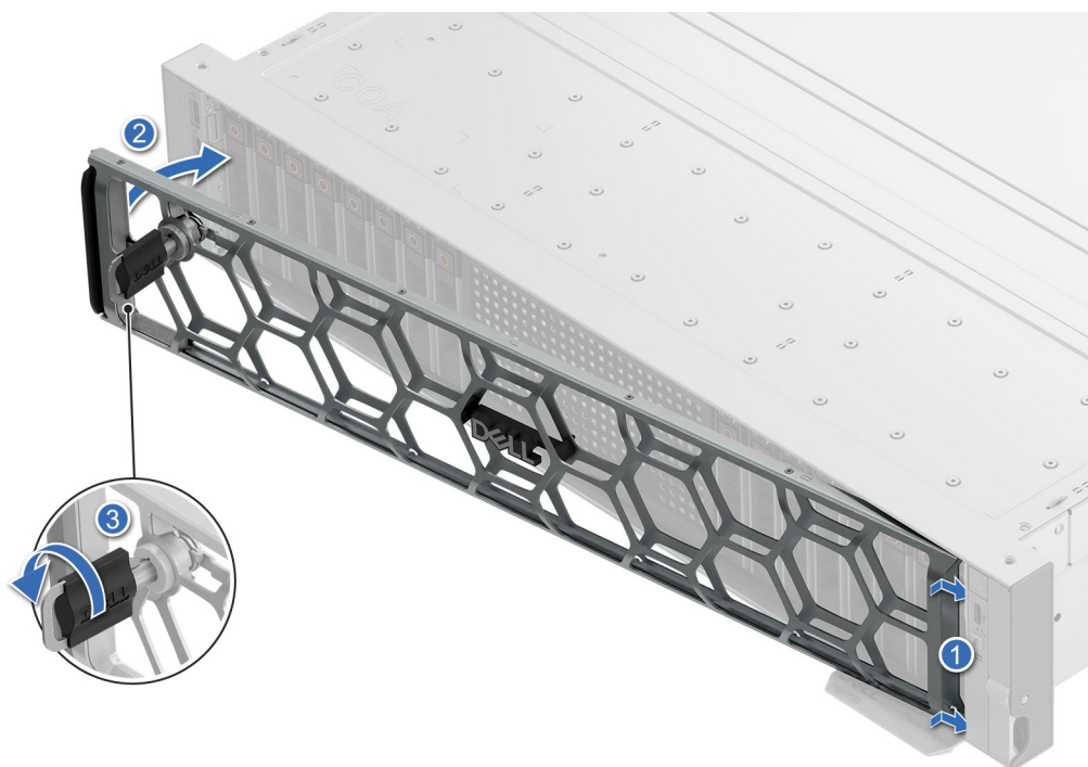
Ilustración 31. Instalación del bisel frontal
