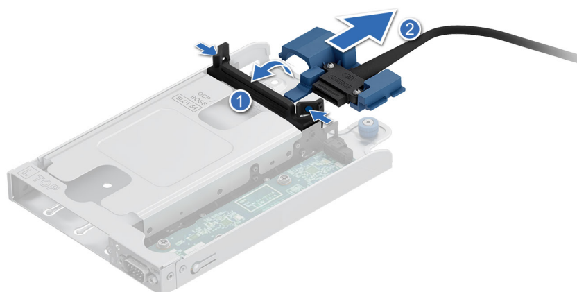
Ilustración 217. Extracción de un cable BOSS-N1 DC-MHS
