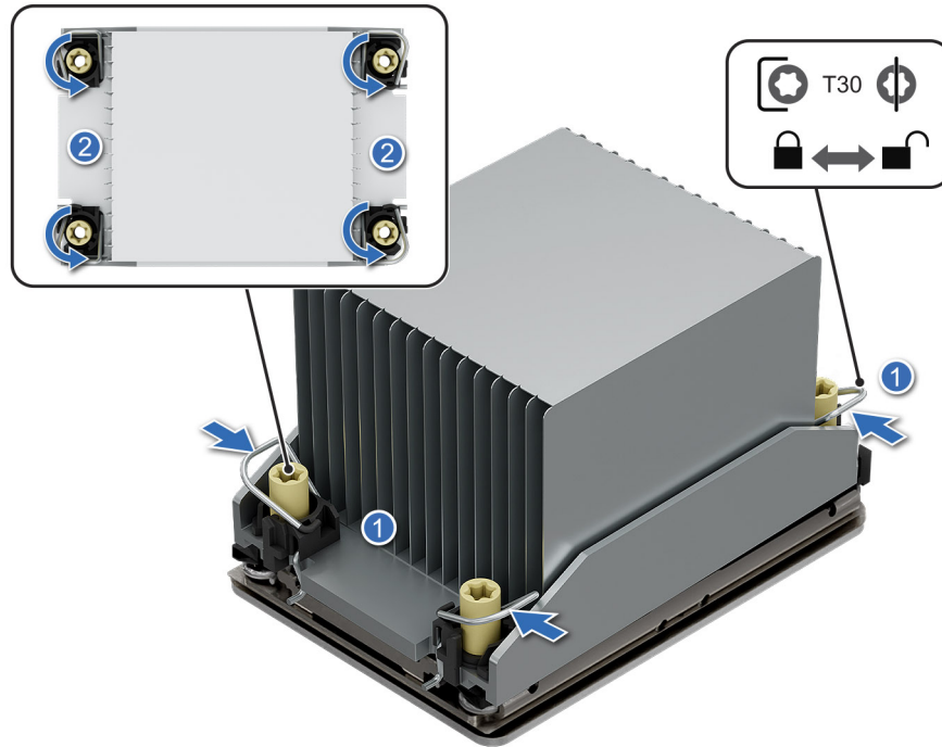
Ilustración 109. Extracción del módulo de disipador de calor del procesador.
