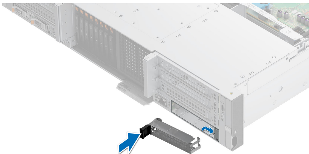
Ilustración 231. Instalación de un soporte de relleno de tarjeta NIC de OCP
