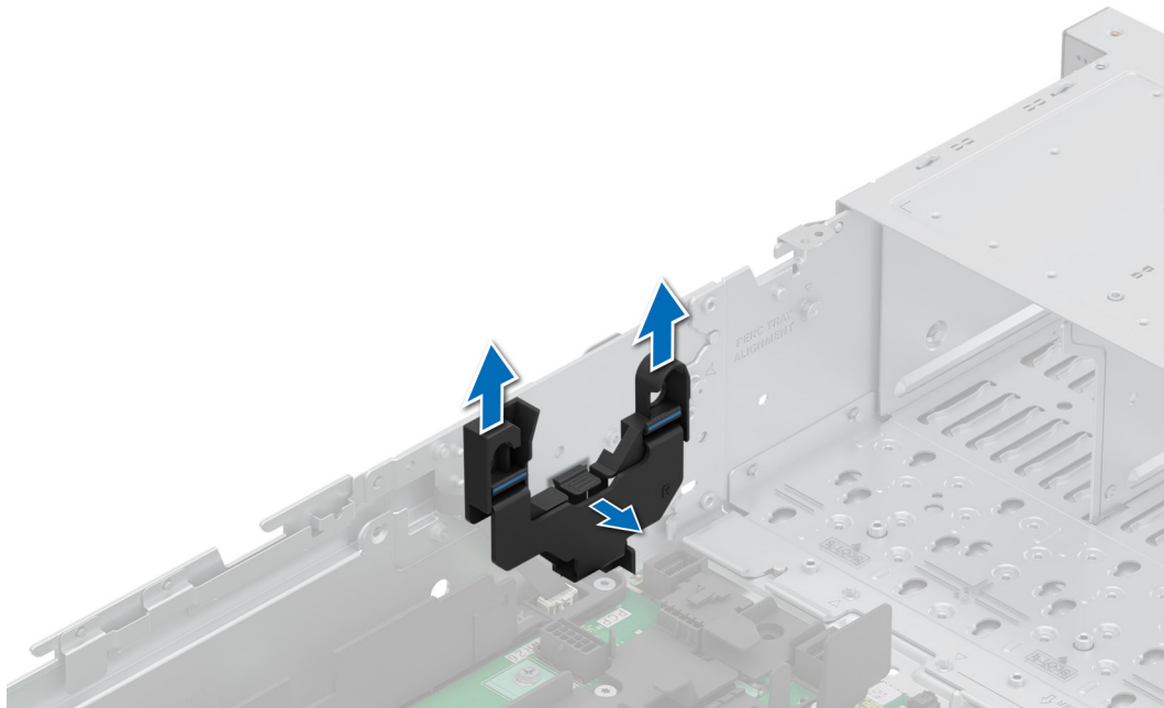
Ilustración 75. Extracción del soporte de pared lateral
