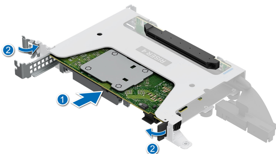
Ilustración 167. Instalación de una tarjeta de expansión en la tarjeta elevadora 4
