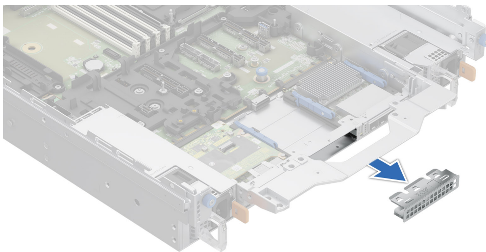
Ilustración 226. Extracción del soporte de relleno
