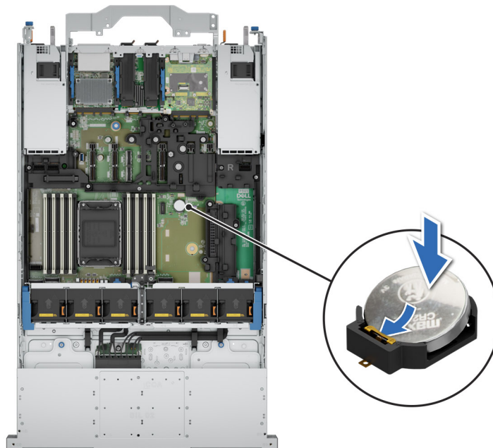
Ilustración 248. Instalación de la batería del sistema
