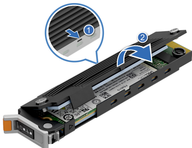
Ilustración 187. Instalación de la cubierta superior
