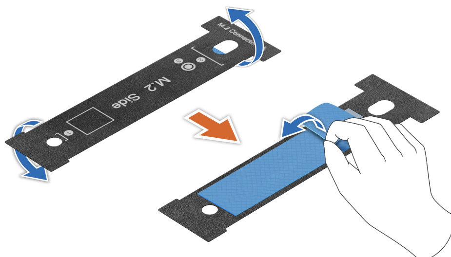
Ilustración 209. Extracción de la película azul de la nueva almohadilla térmica
