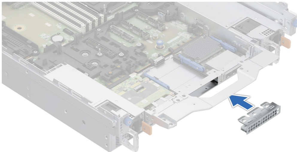
Ilustración 225. Instalación del soporte de relleno
