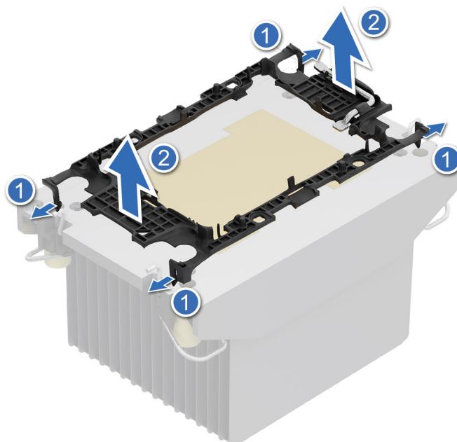
Ilustración 112. Extracción del gancho de retención
