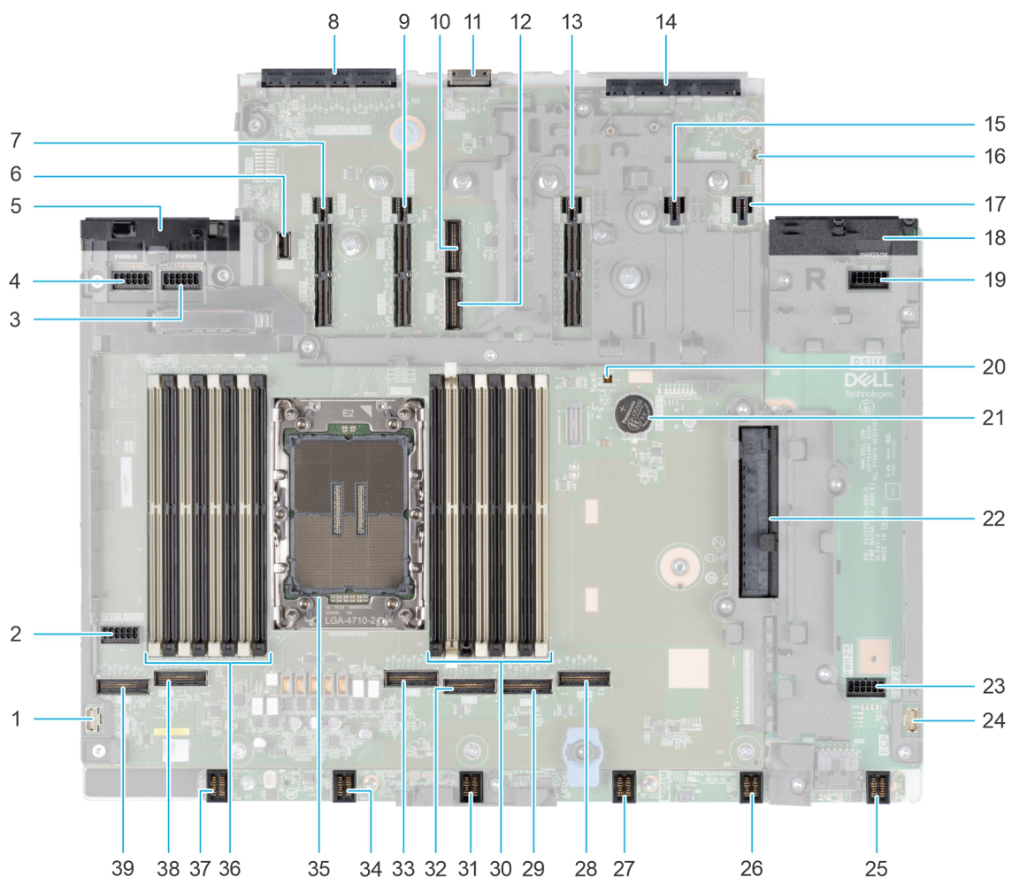
Ilustración 276. Puentes y conectores de la tarjeta madre de HPM
