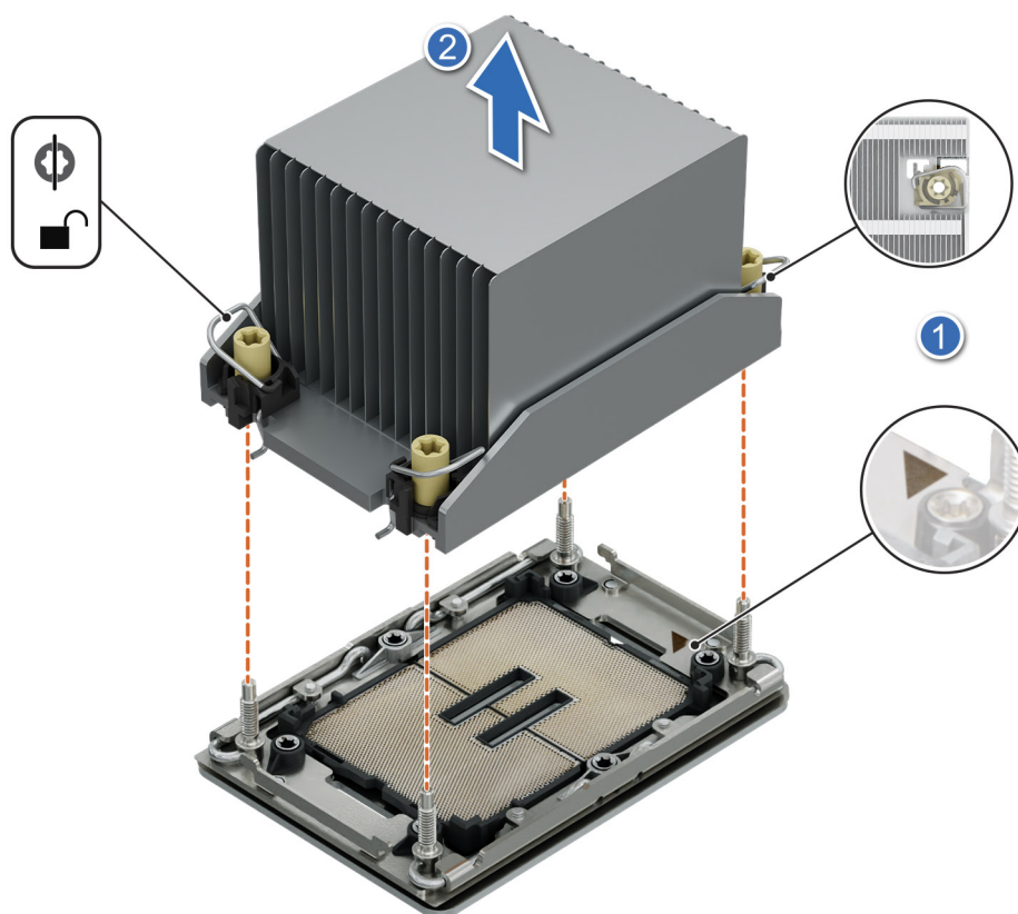
Ilustración 110. Extracción de un disipador de calor
